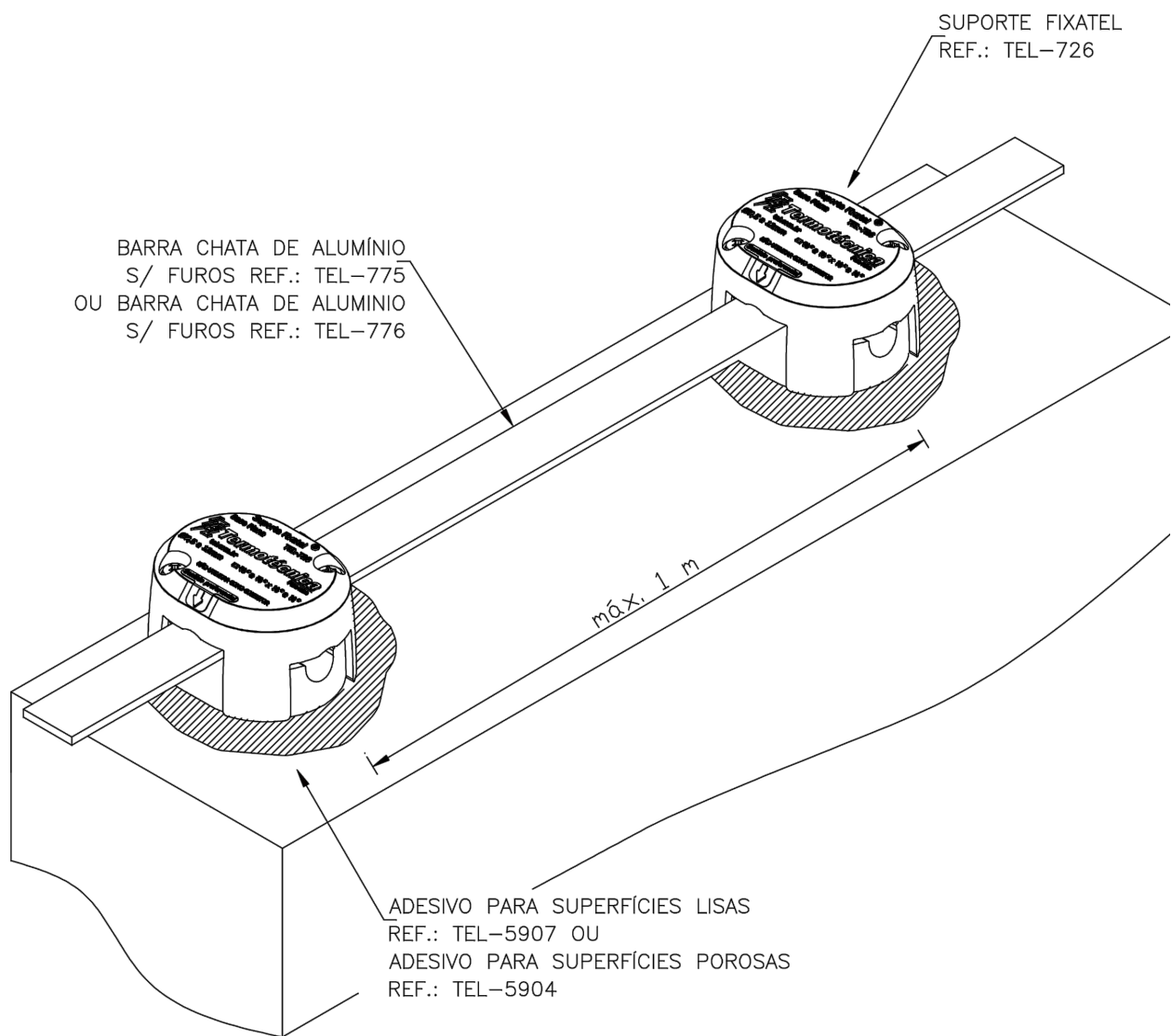
DETALHE - FIXAÇÃO DE BARRA CHATA EM ALUMÍNIO SEM PERFURAÇÃO SEM ESCALA
