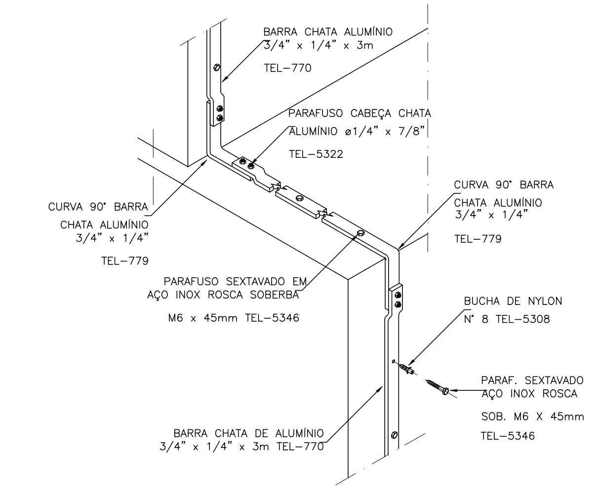
DETALHE - DESCIDA DE BARRA CHATA PELA PAREDE SEM ESCALA
