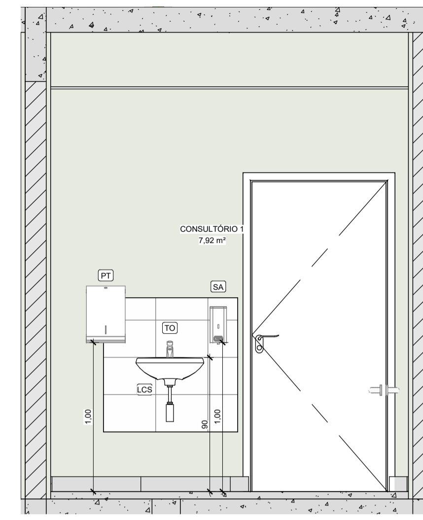
2 DET. CONSULTÓRIO 1 (1) 1 : 25
