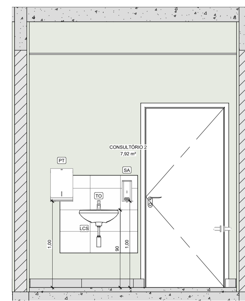
3 DET. CONSULTÓRIO 2 (1) 1 : 25
