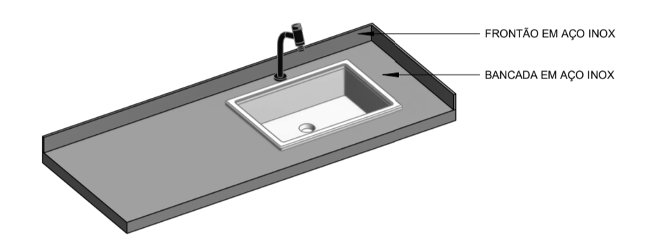
6 DET - BANCADA INOX 1:20
