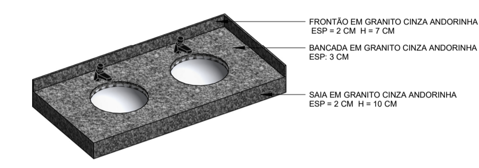
5 DET - BANCADA GRANITO 1:20
