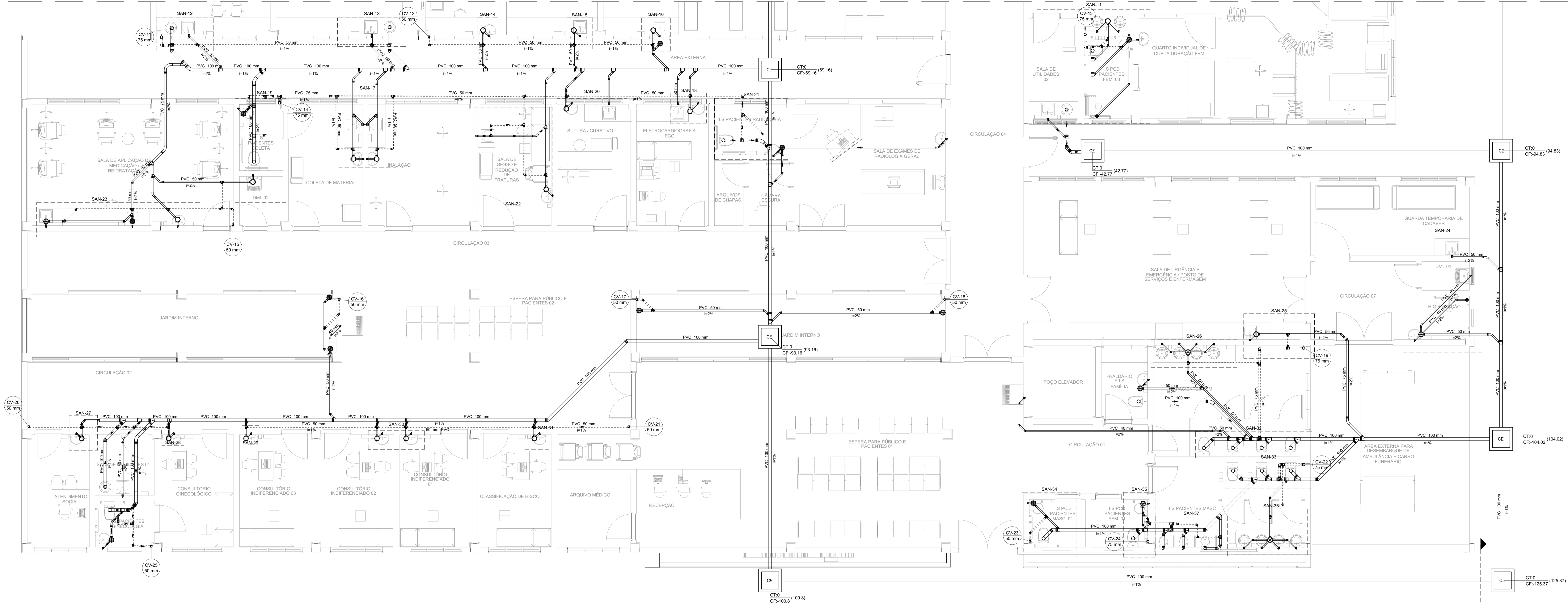
PLANTA BAIXA - TÉRREO - PARTE 2 ESCALA 1:50
