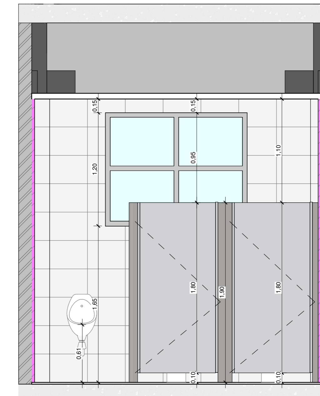
5 DETALHE 2 - I.S. MASCULINO 1 1 : 25
