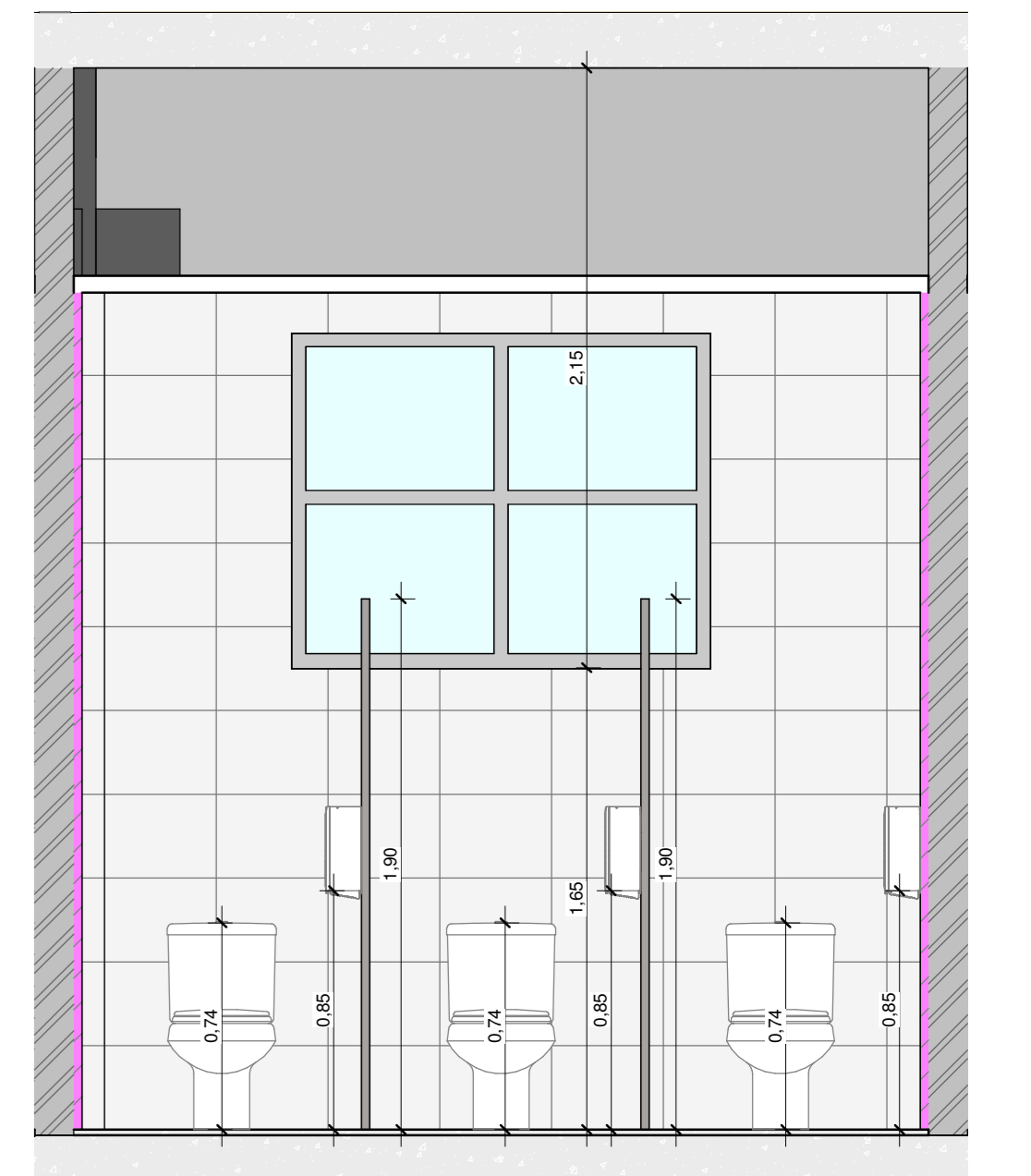
12 DETALHE 3 - I.S. FEMININO 1 1 : 25
