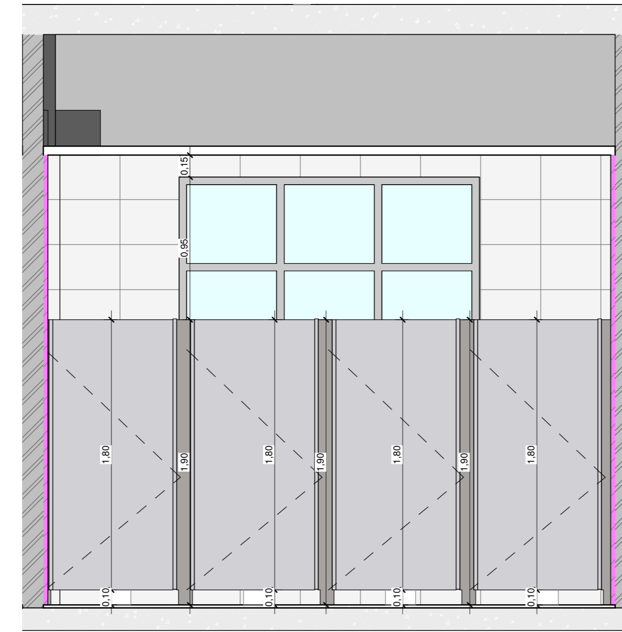
16 DETALHE 2 - I.S. FEMININO 2 1 : 25
