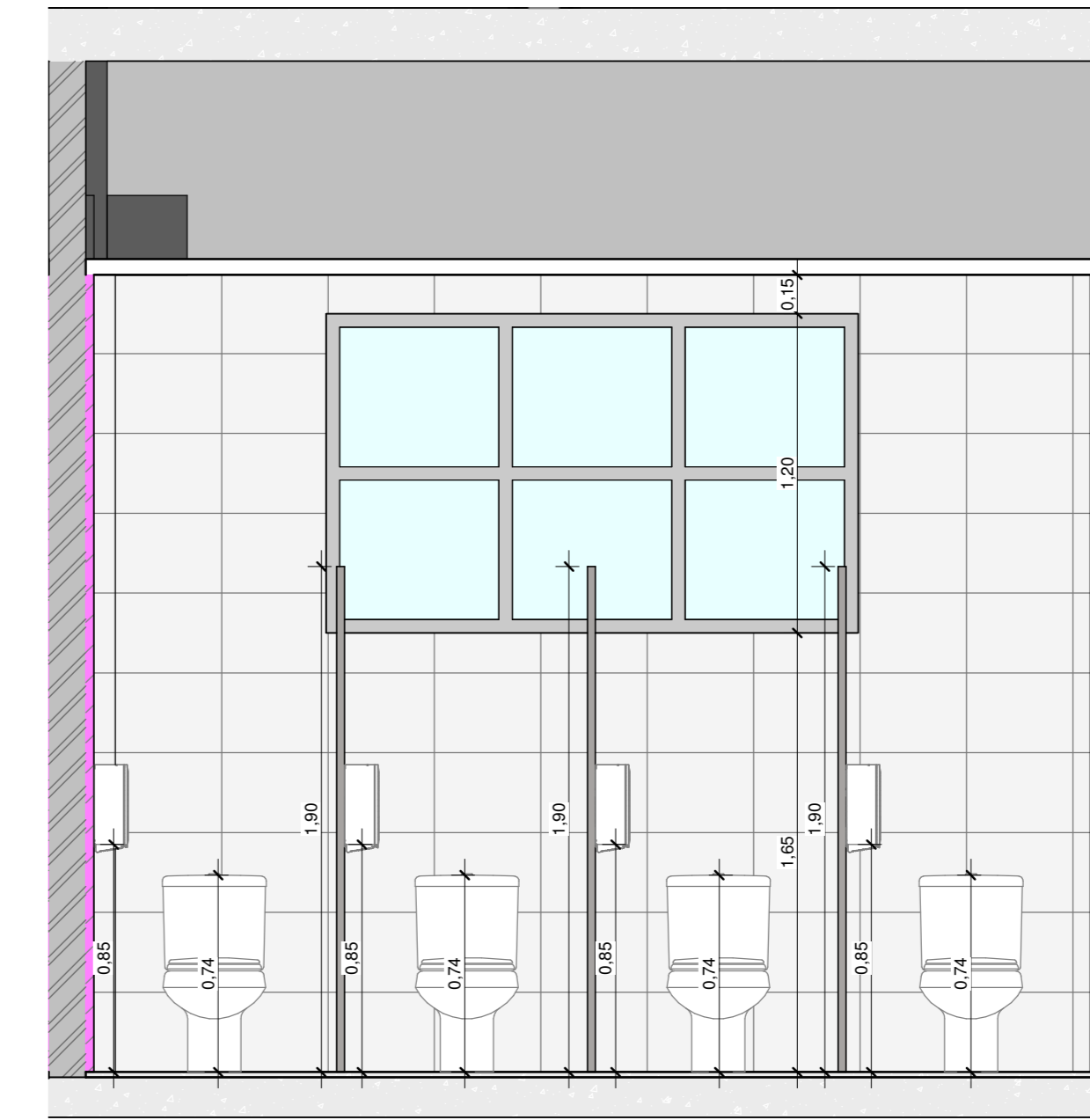
17 DETALHE 3 - I.S. FEMININO 2 1 : 25
