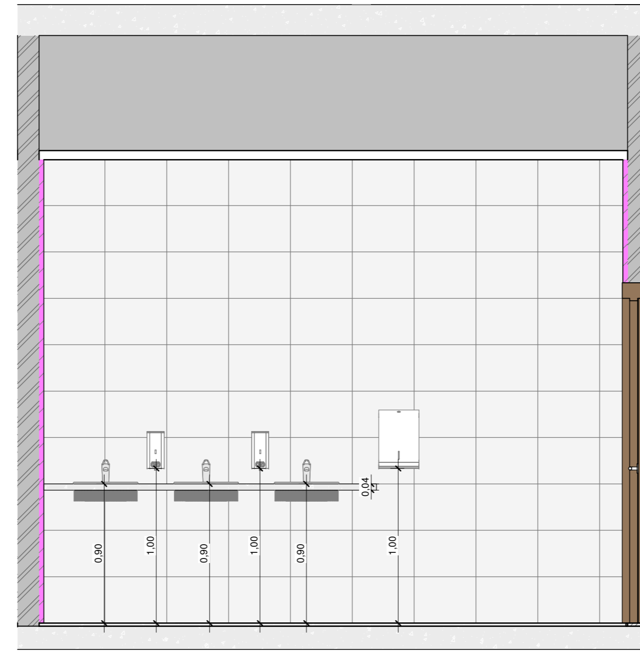
15 DETALHE 1 - I.S. FEMININO 2 1 : 25
