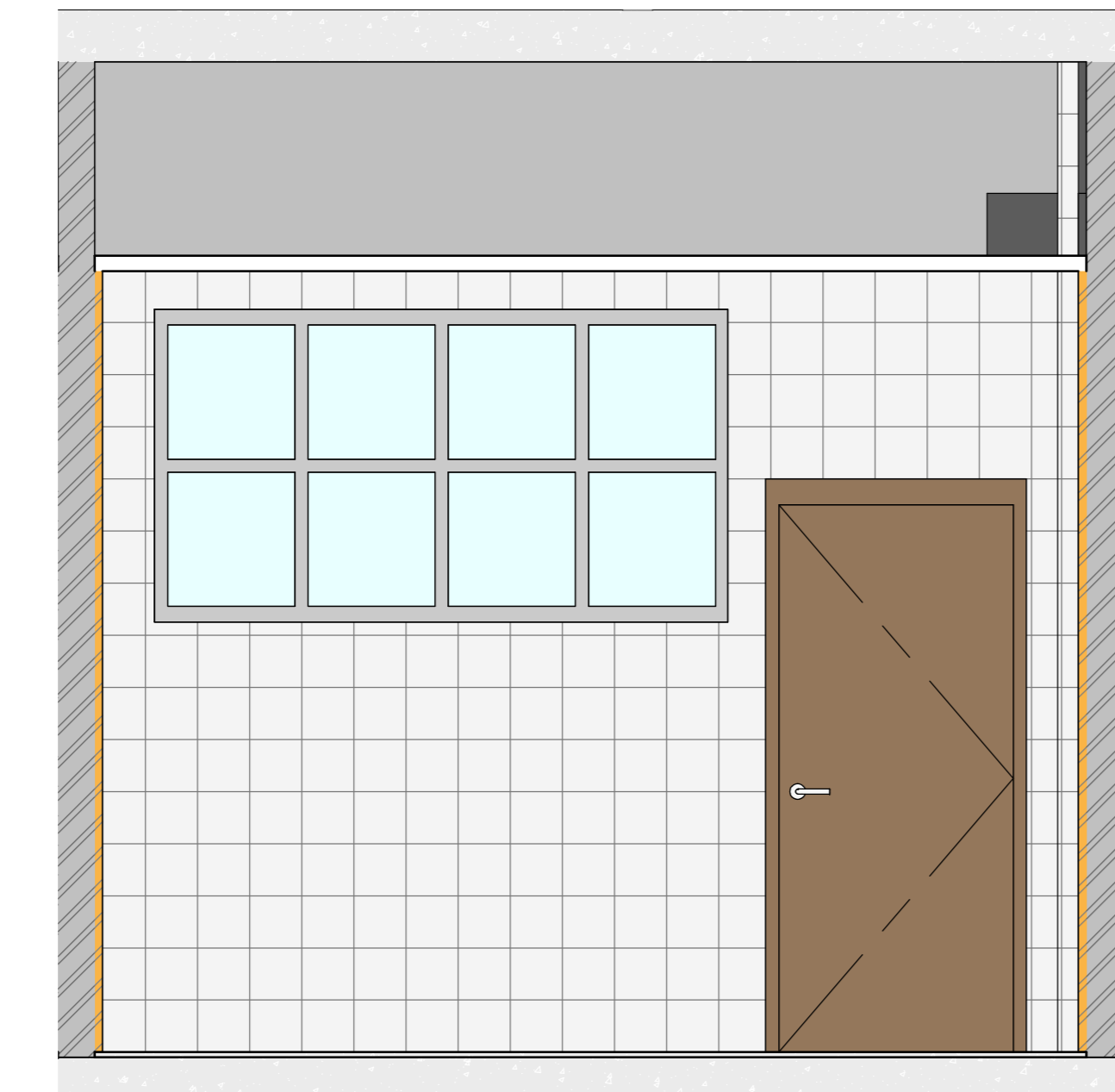
8 DETALHE COPA FUNCIONÁRIOS 1 : 25
