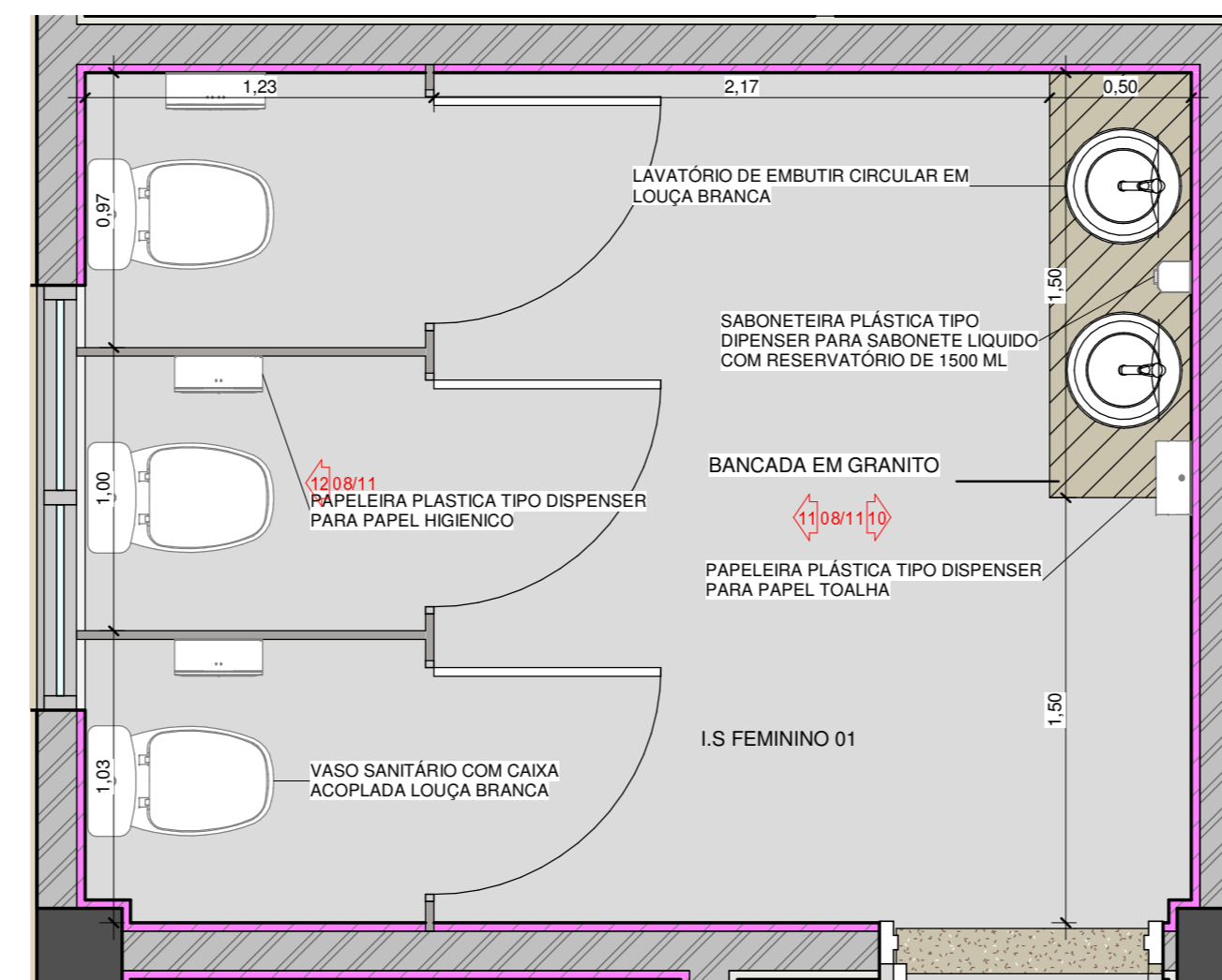
9 DETALHE I.S. FEMININO 1 1 : 25
