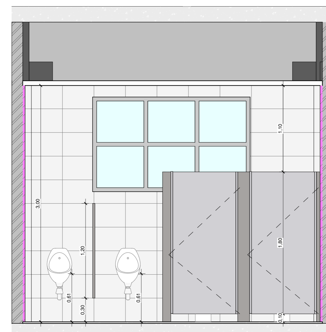
21 DETALHE 2 - I.S. MASCULINO 2 1 : 25
