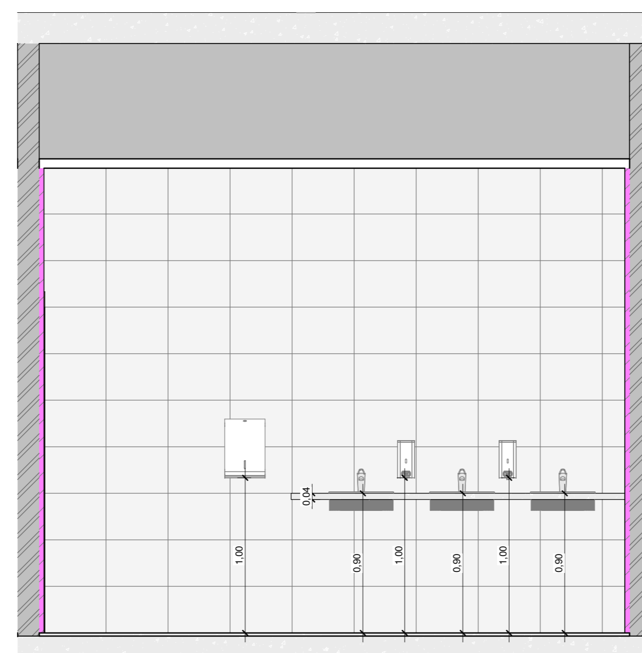
20 DETALHE 1 - I.S. MASCULINO 2 1 : 25
