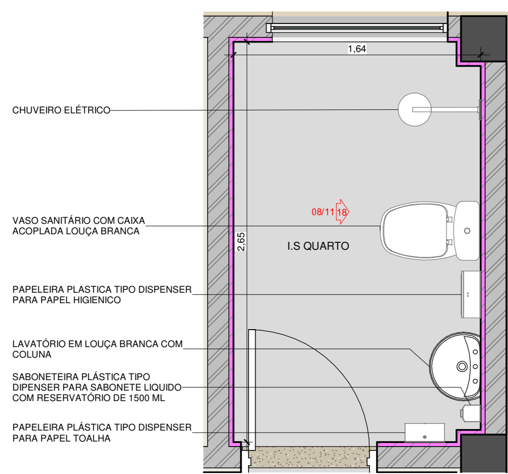
13 DETALHE I.S. QUARTO 1 : 25
