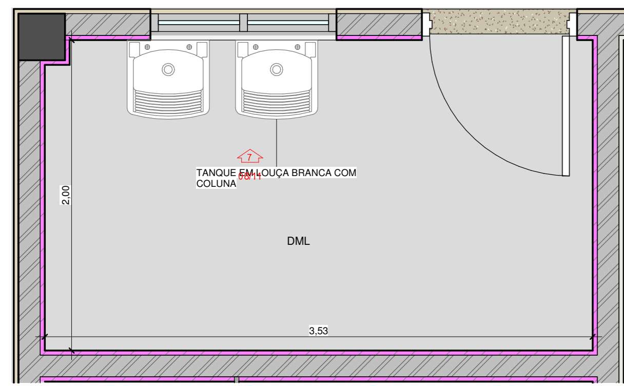
1 DETALHE DML 1 : 25
