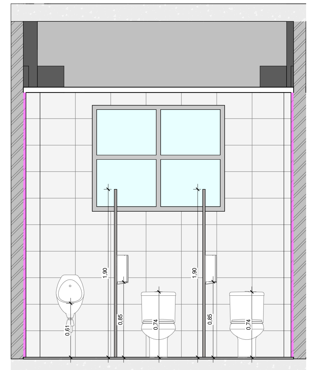
6 DETALHE 3 - I.S. MASCULINO 1 1 : 25
