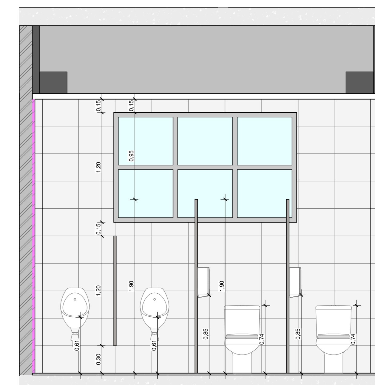
22 DETALHE 3 - I.S. MASCULINO 2 1 : 25
