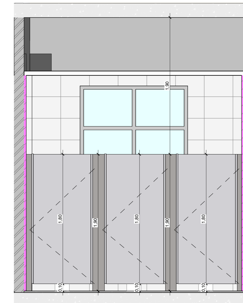
11 DETALHE 2 - I.S. FEMININO 1 1 : 25
