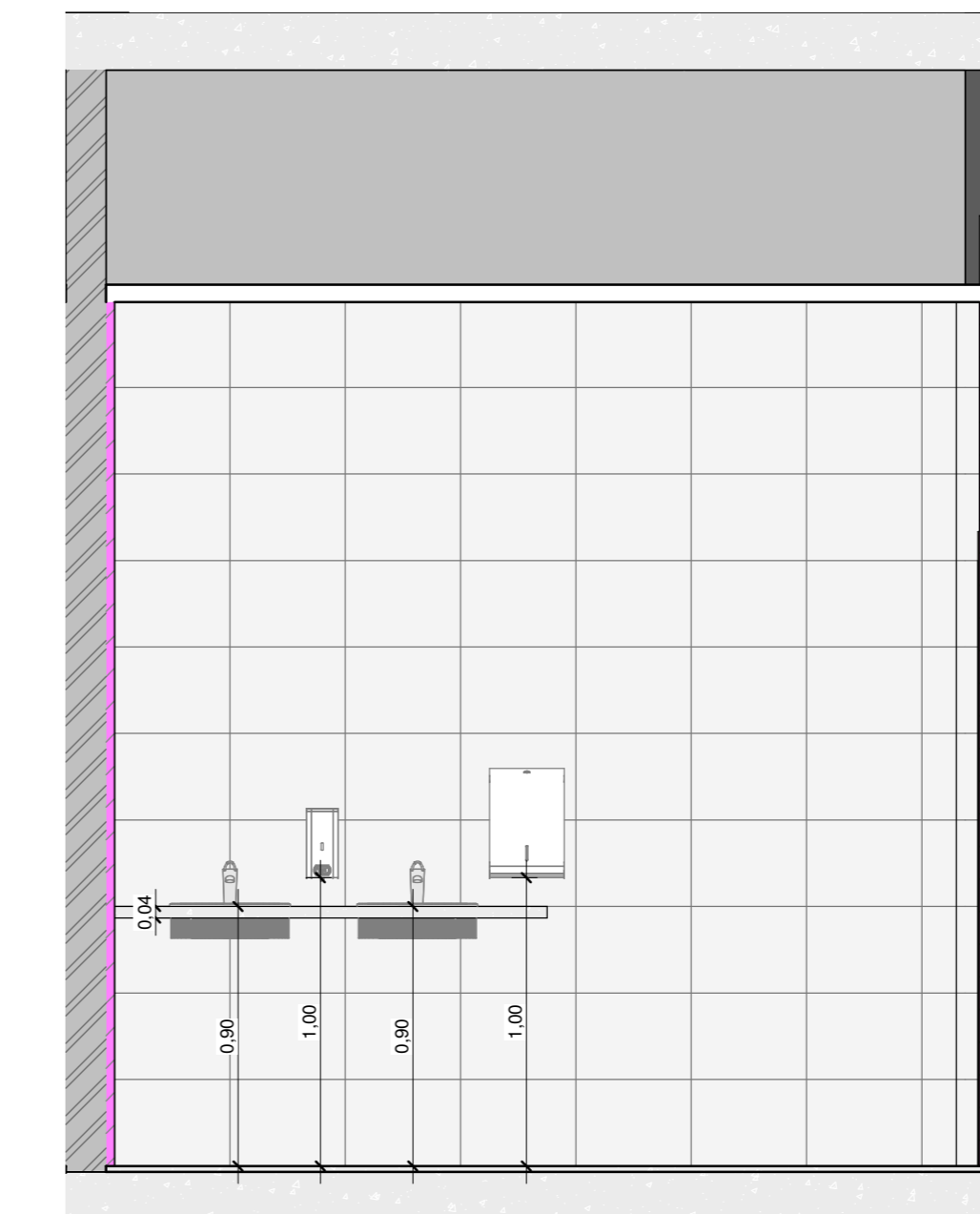
10 DETALHE 1 - I.S. FEMININO 1 1 : 25
