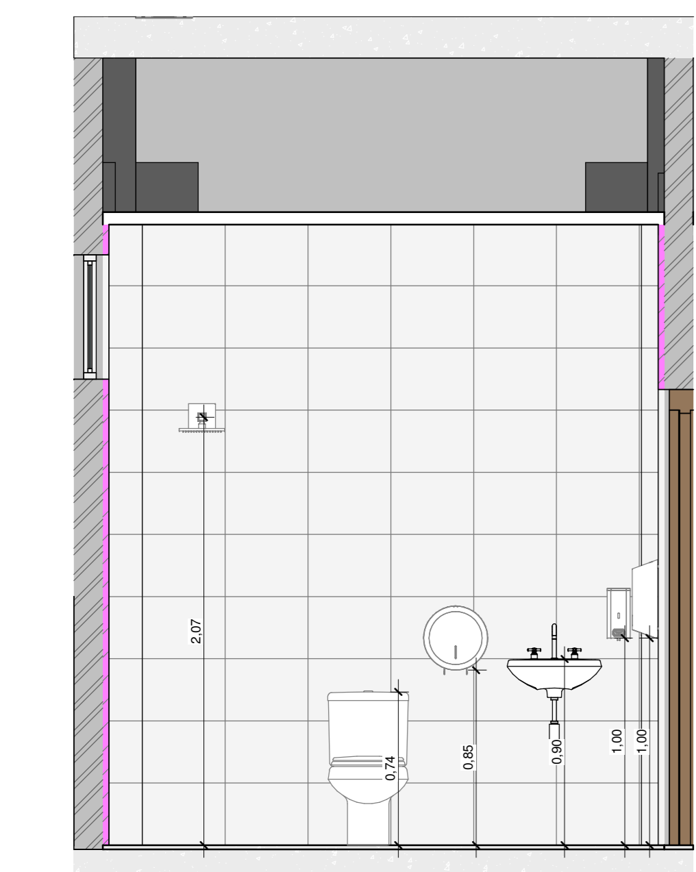
18 DETALHE I.S. QUARTO 1 : 25
