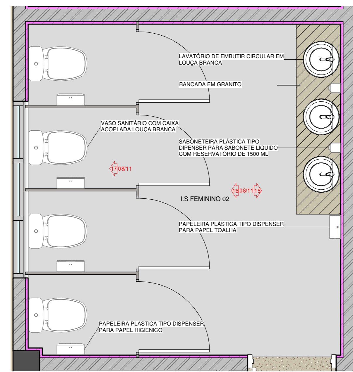
14 DETALHE I.S. FEMININO 2 1 : 25
