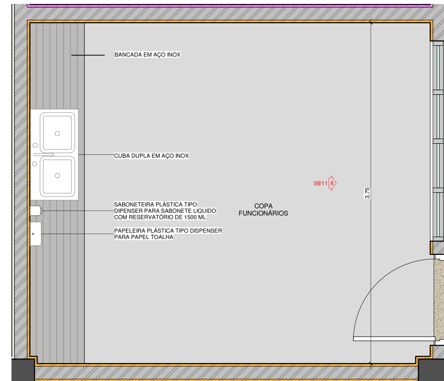
2 DETALHE COPA FUNCIONÁRIOS 1 : 25
