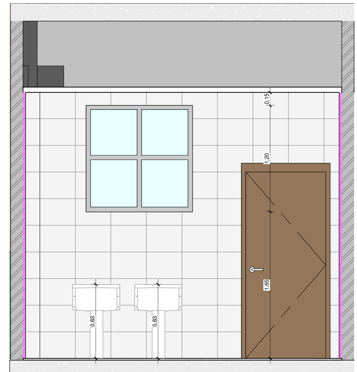
7 DETALHE DML 1 : 25
