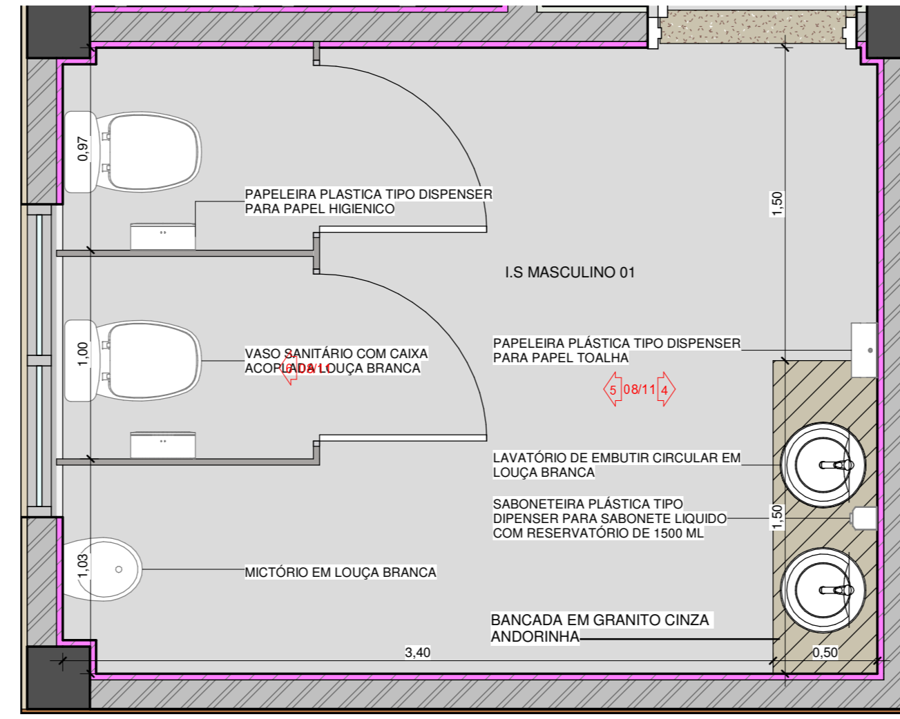
3 DETALHE I.S. MASCULINO 1 1 : 25
