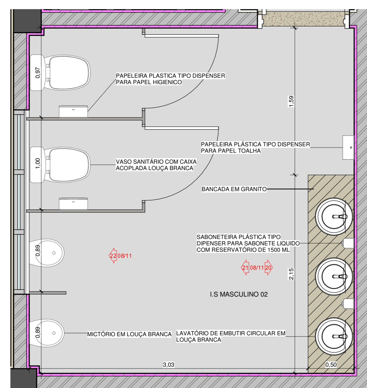
19 DETALHE I.S. MASCULINO 2 1 : 25
