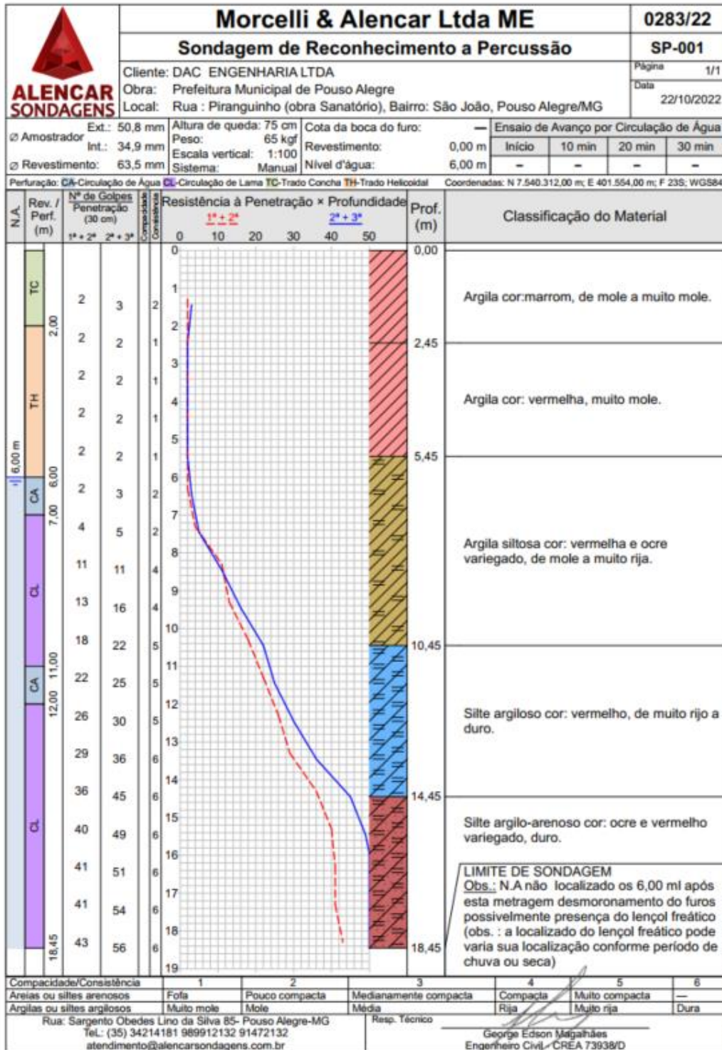
Figura 5-2 – Laudo de Sondagem
