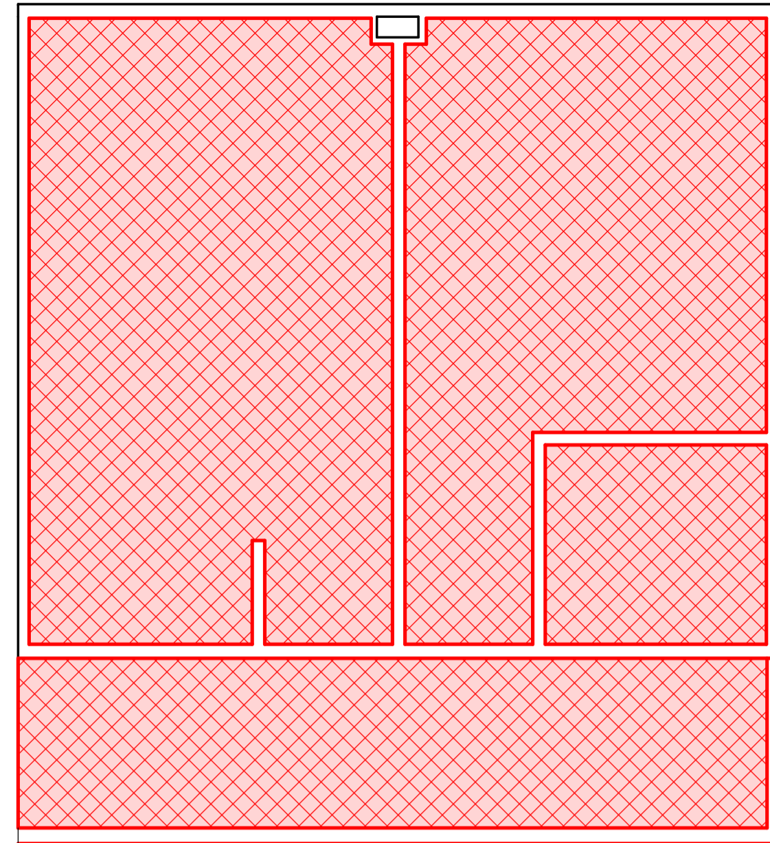
3 PLANTA DE IMPERMEABILIZAÇÃO SUPERIOR 1 : 50
