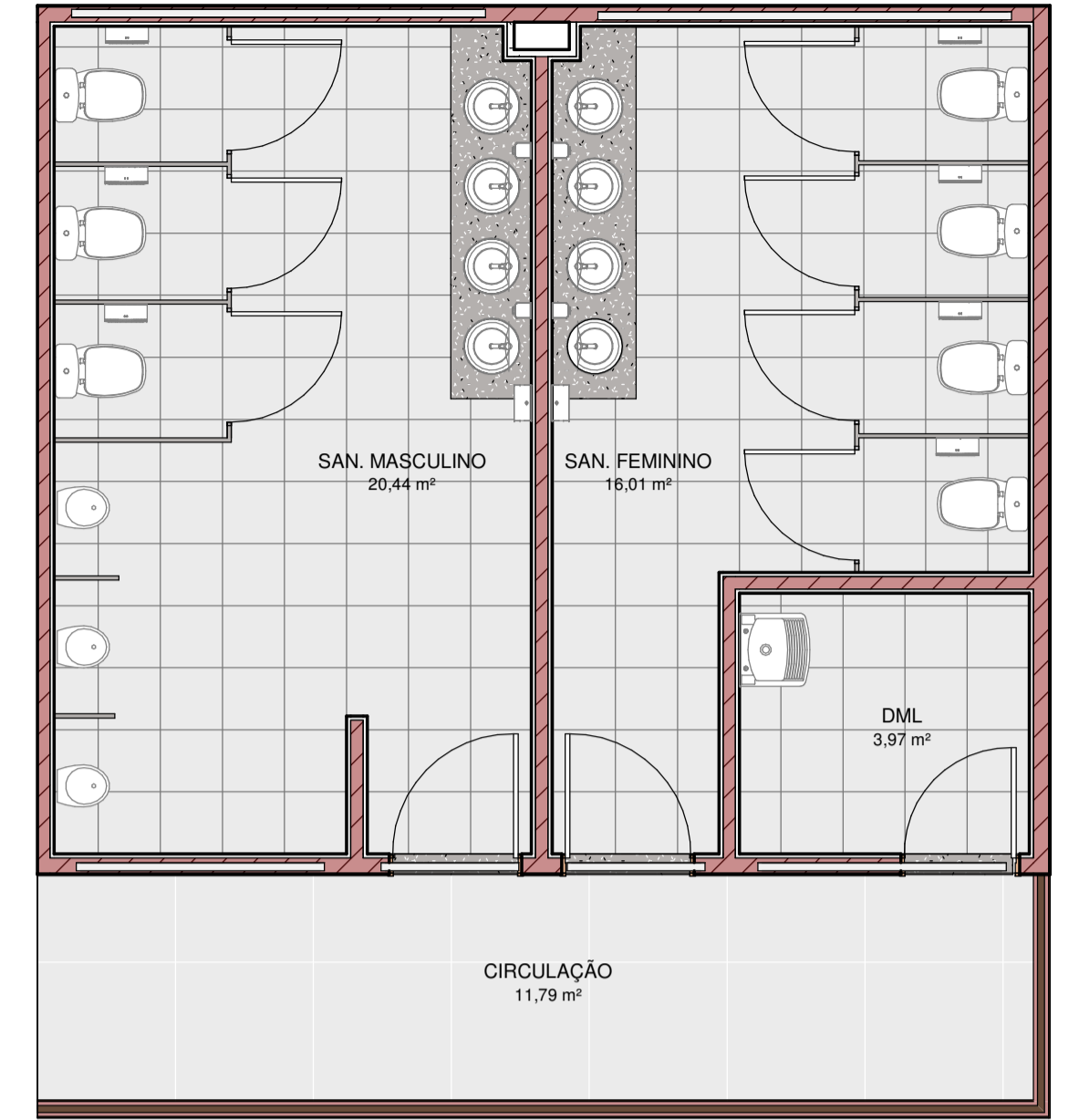
7 PLANTA DE LAYOUT SUPERIOR 1 : 50
