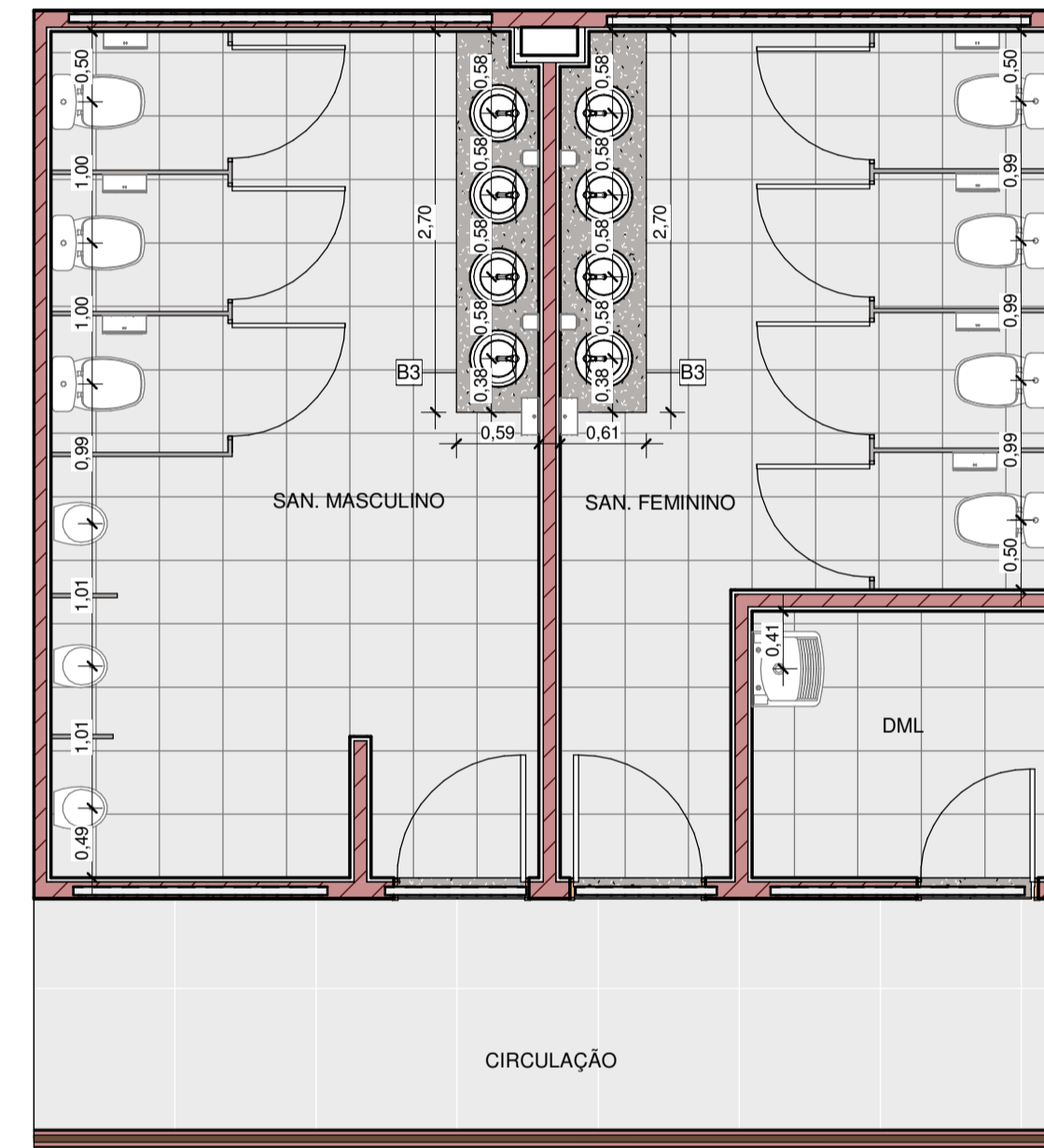
6 PLANTA DE EIXO HIDRAULICO PAV. SUPERIOR 1 : 50
