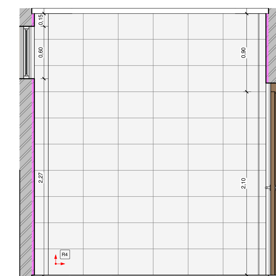
17 VISTA 2 - I.S QUARTO 1:25
