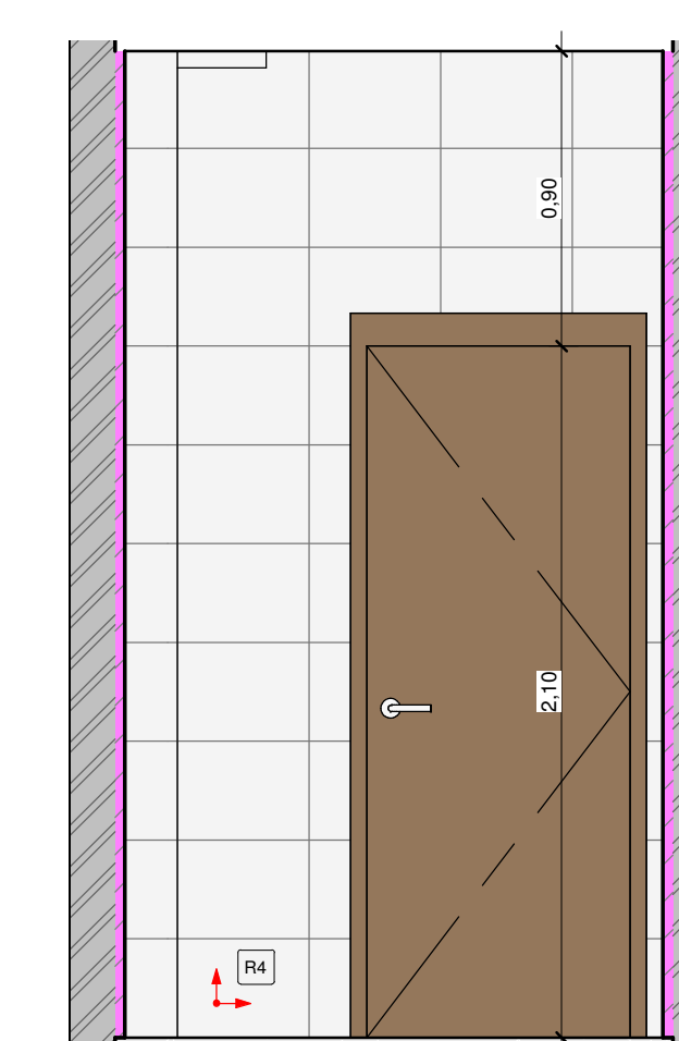
18 VISTA 3 - I.S QUARTO 1:25
