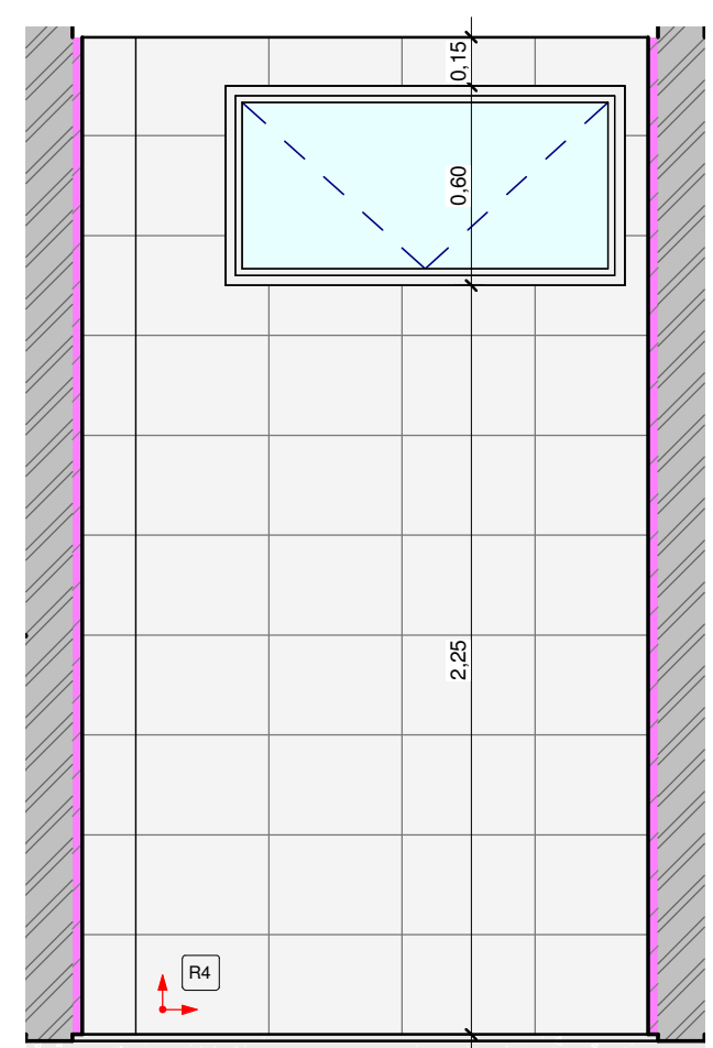
5 VISTA 4 - I.S PNE MASC 03 1:25
