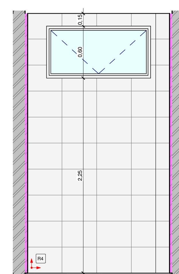
16 VISTA 1 - I.S QUARTO 1:25
