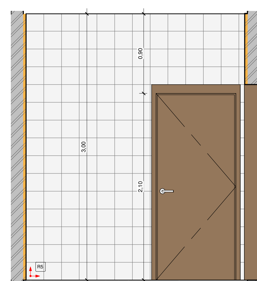
15 VISTA 4 - TRIAGEM 1:25
