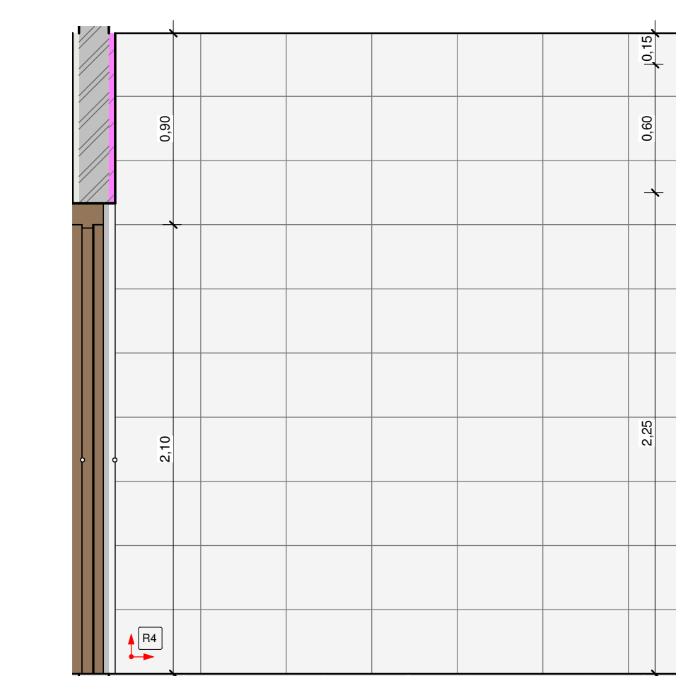
19 VISTA 4 - I.S QUARTO 1:25
