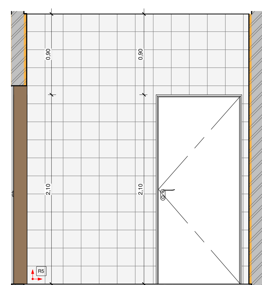
13 VISTA 2 - TRIAGEM 1:25
