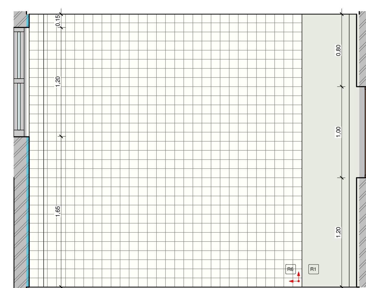
11 VISTA 2 - SERVIÇOS E ENFERMAGEM 1:25
