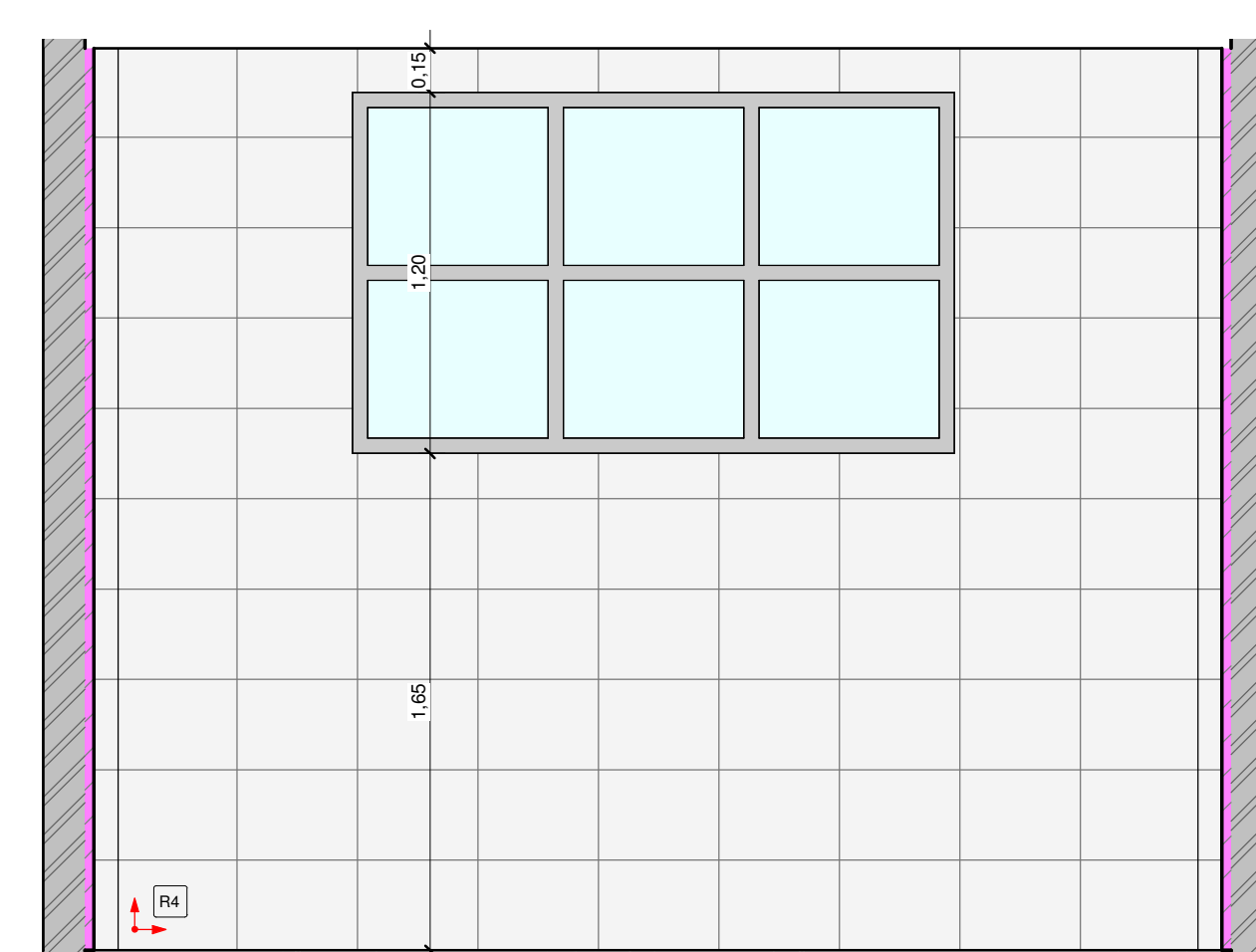
23 VISTA 4 - I.S MASCULINO 02 1:25
