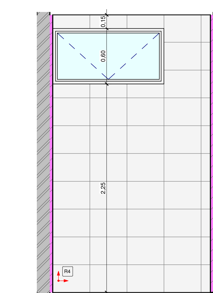
27 VISTA 4 - I.S PNE FEM 03 1:25
