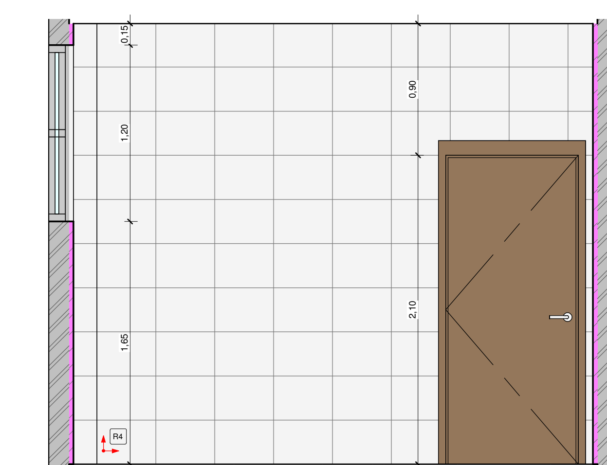
20 VISTA 1 - I.S MASCULINO 02 1:25
