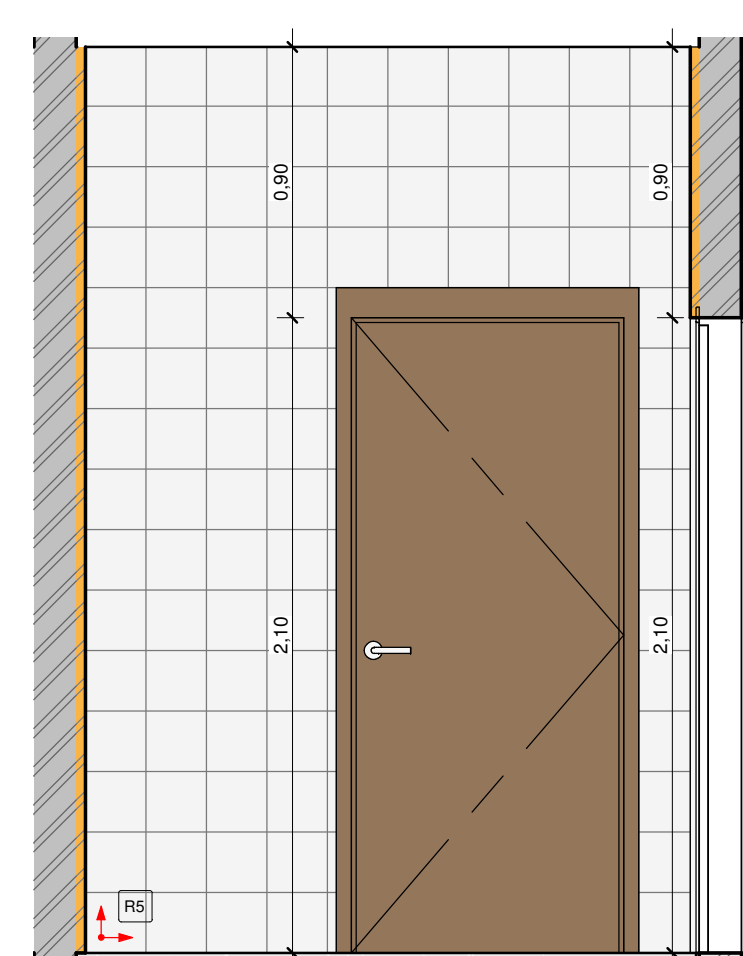
12 VISTA 1 - TRIAGEM 1:25
