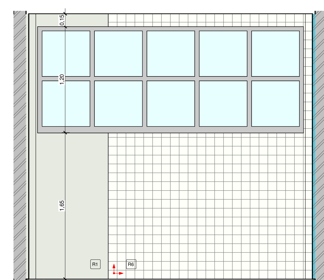
10 VISTA 1 - SERVIÇOS E ENFERMAGEM 1:25
