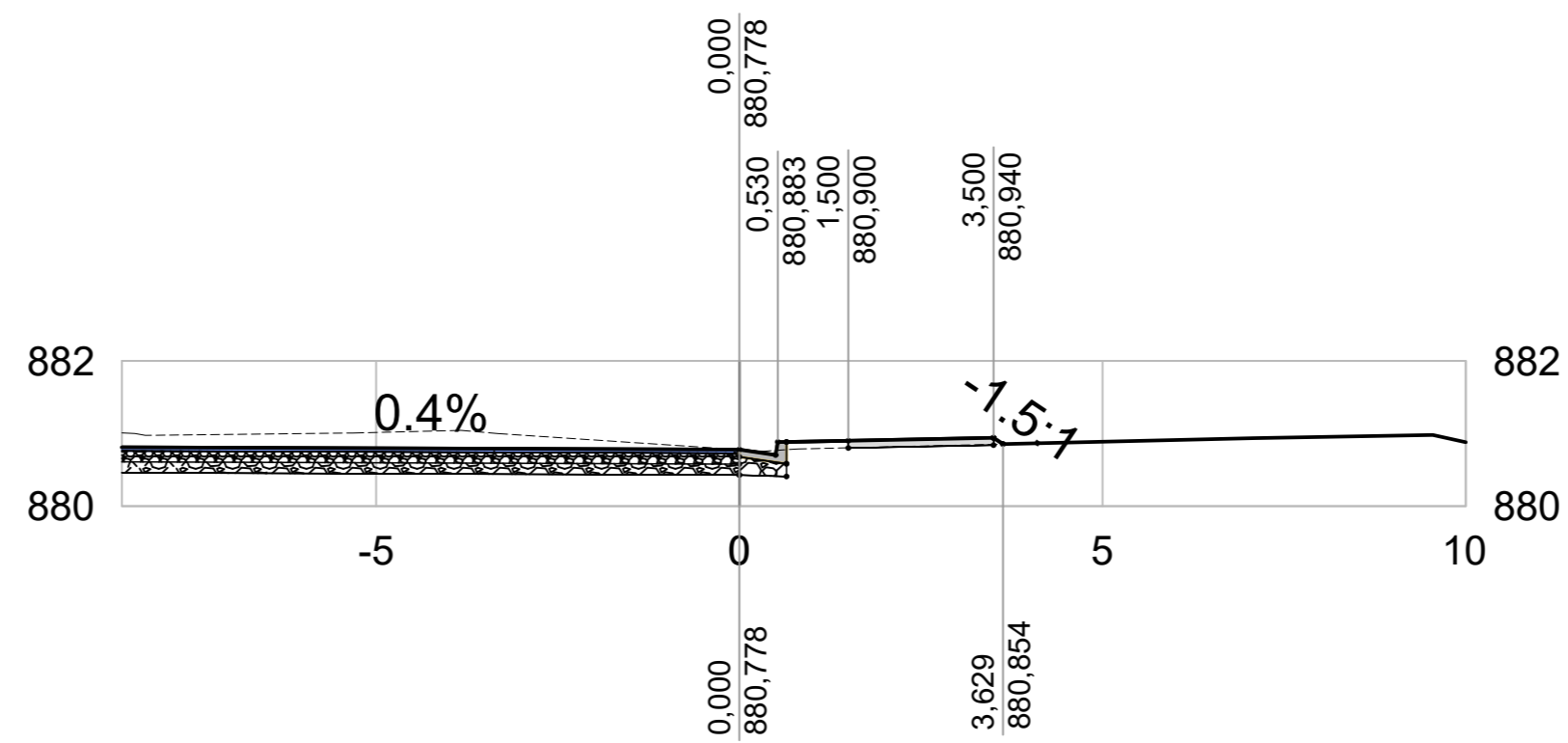
RAMO 400 - EST. 5+19,22m
