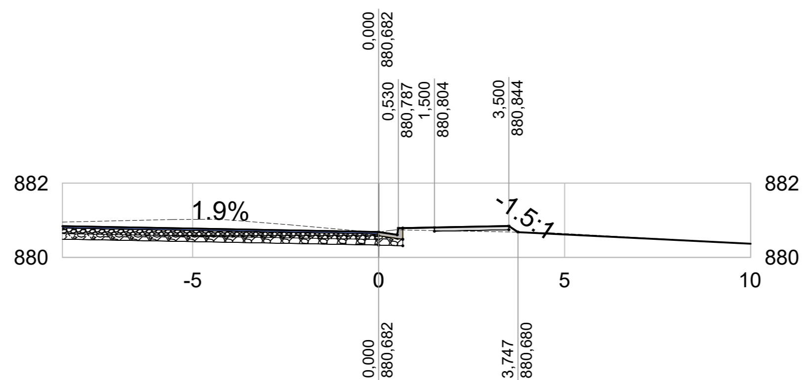
RAMO 400 - EST. 5+0,00m
