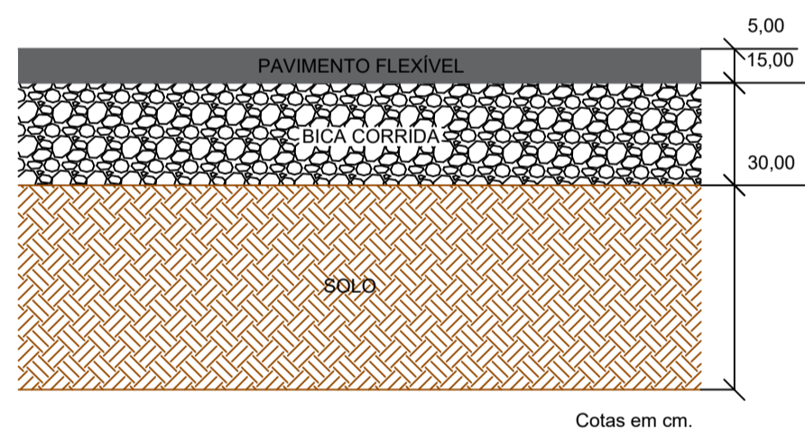
DETALHE 01 - DEMOLIÇÃO DE PAVIMENTO FLEXÍVEL 01 SEM ESCALA
