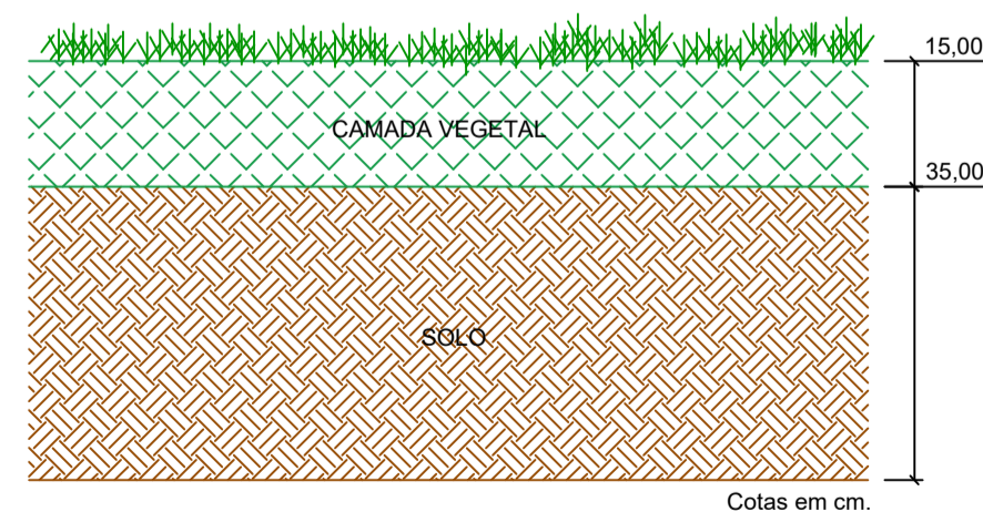
DETALHE 07 - LIMPEZA DA CAMADA VEGETAL 02 SEM ESCALA
