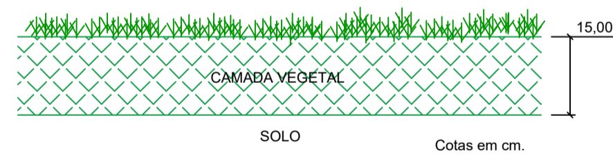
DETALHE 05 - LIMPEZA DA CAMADA VEGETAL 01 SEM ESCALA
