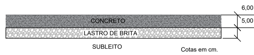
DETALHE 04 - DEMOLIÇÃO DE CALÇADA 01 SEM ESCALA
