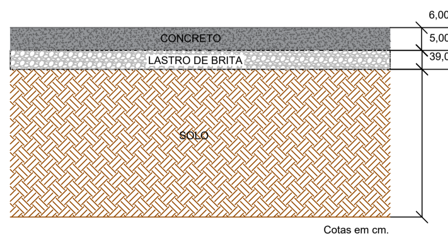
DETALHE 06 - DEMOLIÇÃO DE CALÇADA 02 SEM ESCALA
