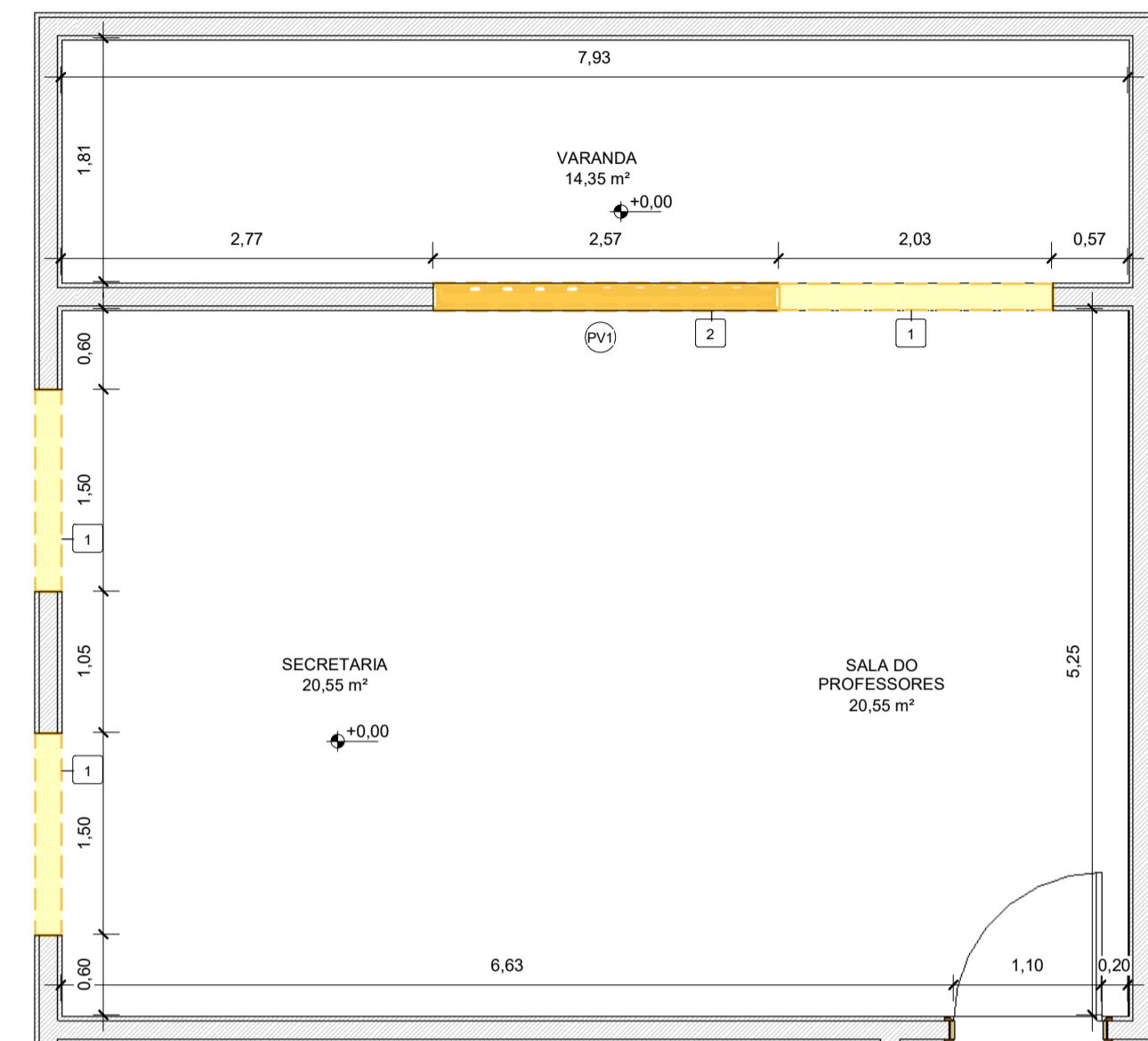
2 PLANTA BAIXA - DEMOLIÇÃO 1 : 50
