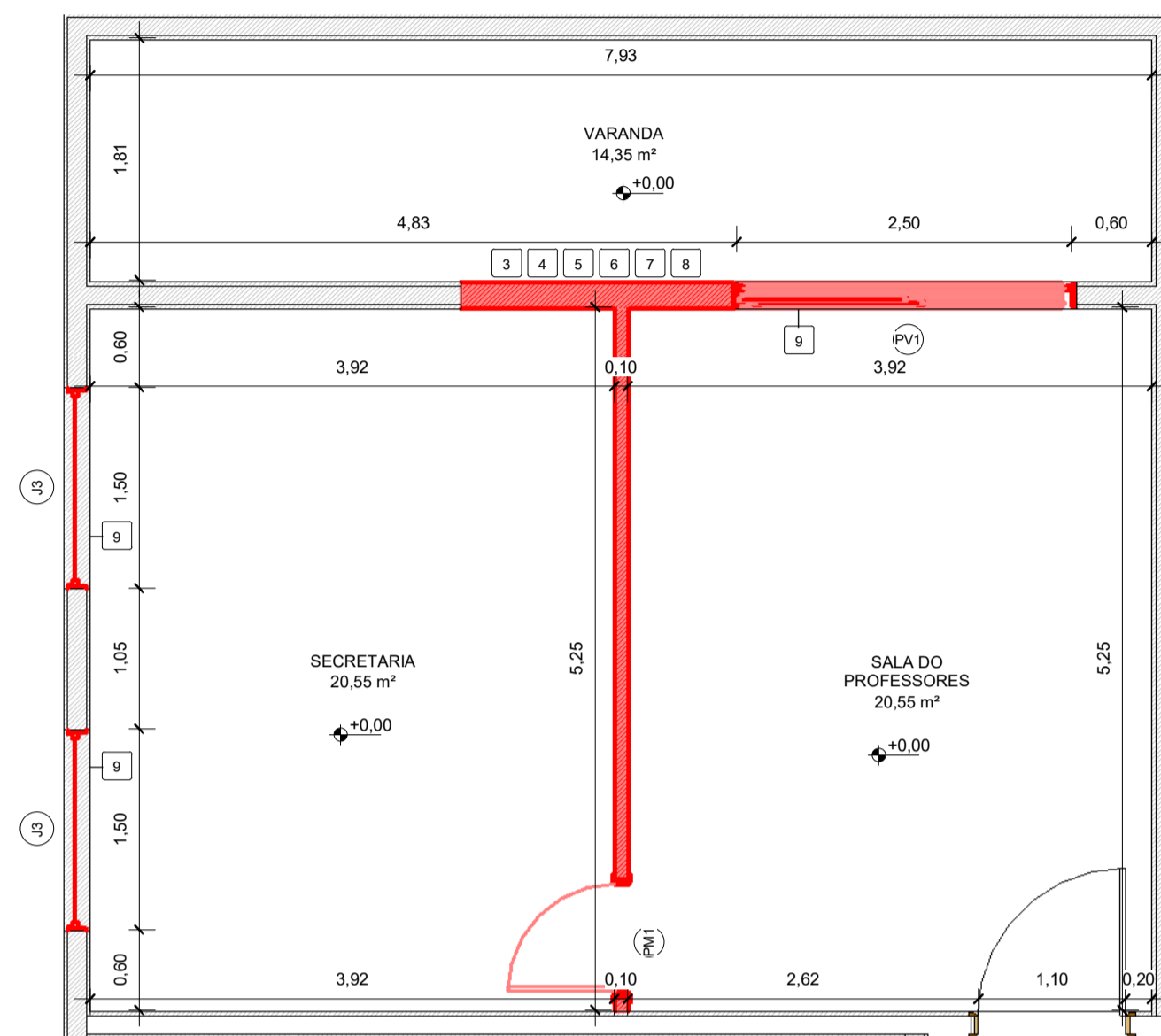
3 PLANTA BAIXA - CONSTRUÇÃO 1 : 50
