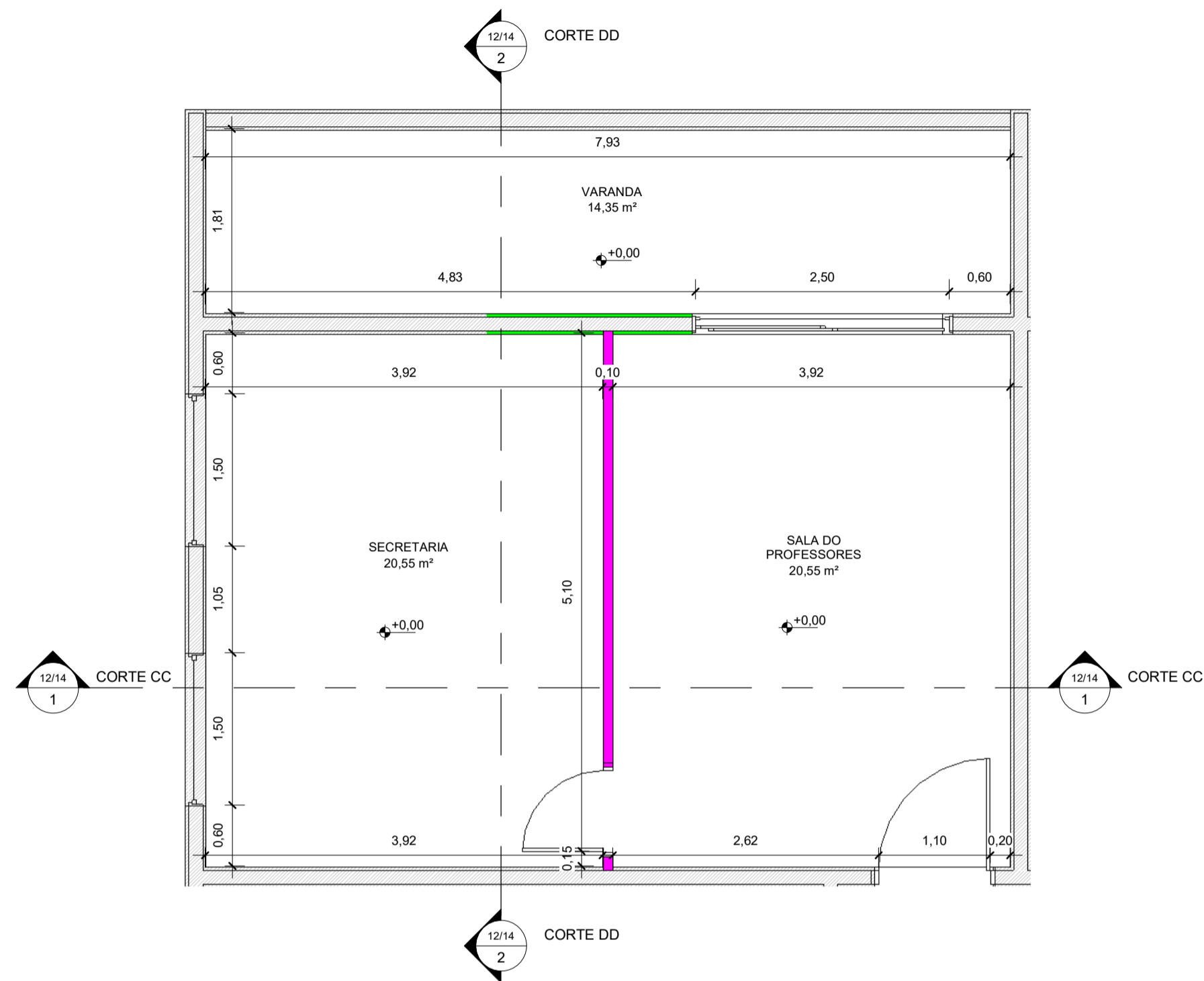
1 PLANTA BAIXA - ESCOLA 1 : 50
