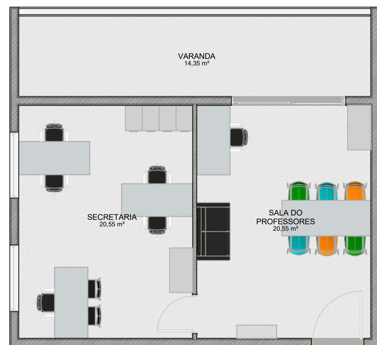
4 PLANTA DE LAYOUT - SECRETARIA / SALA DOS PROFESSORES 1 : 50
