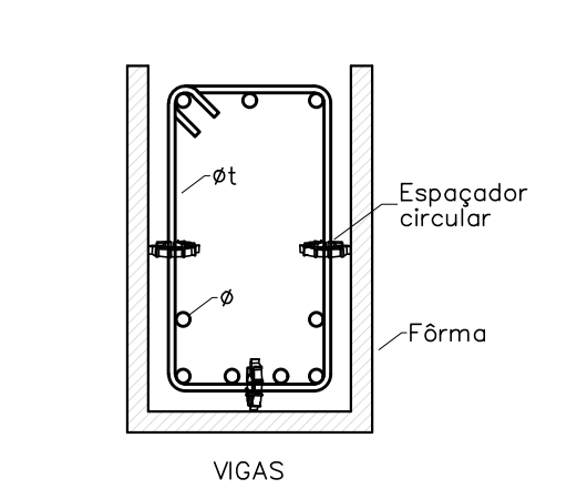
ESPAÇADORES NAS VIGAS SEM ESCALA
