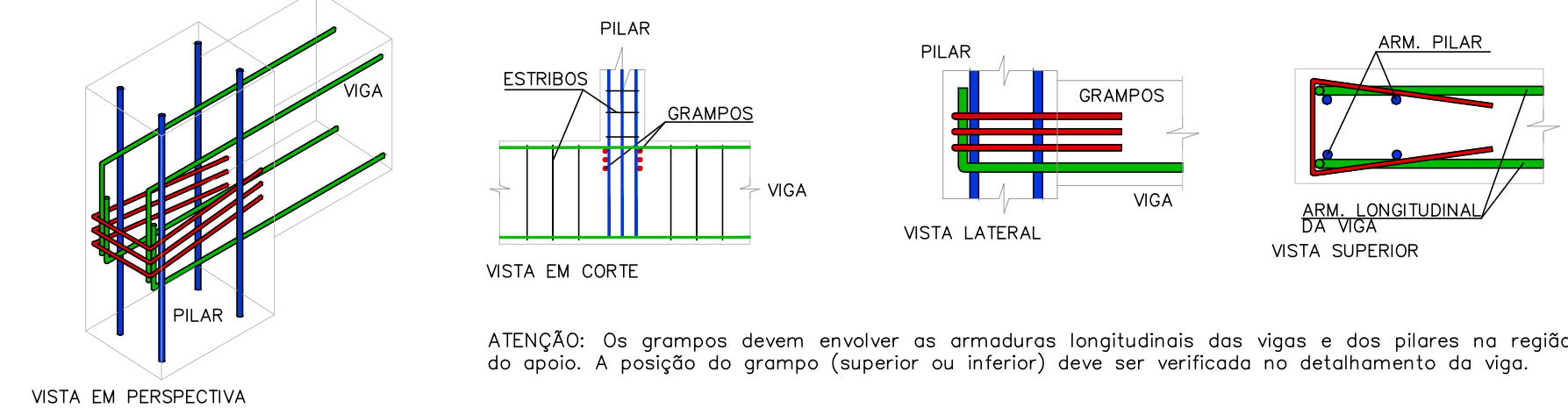
GRAMPOS DE ANCORAGEM – VIGAS SEM ESCALA
