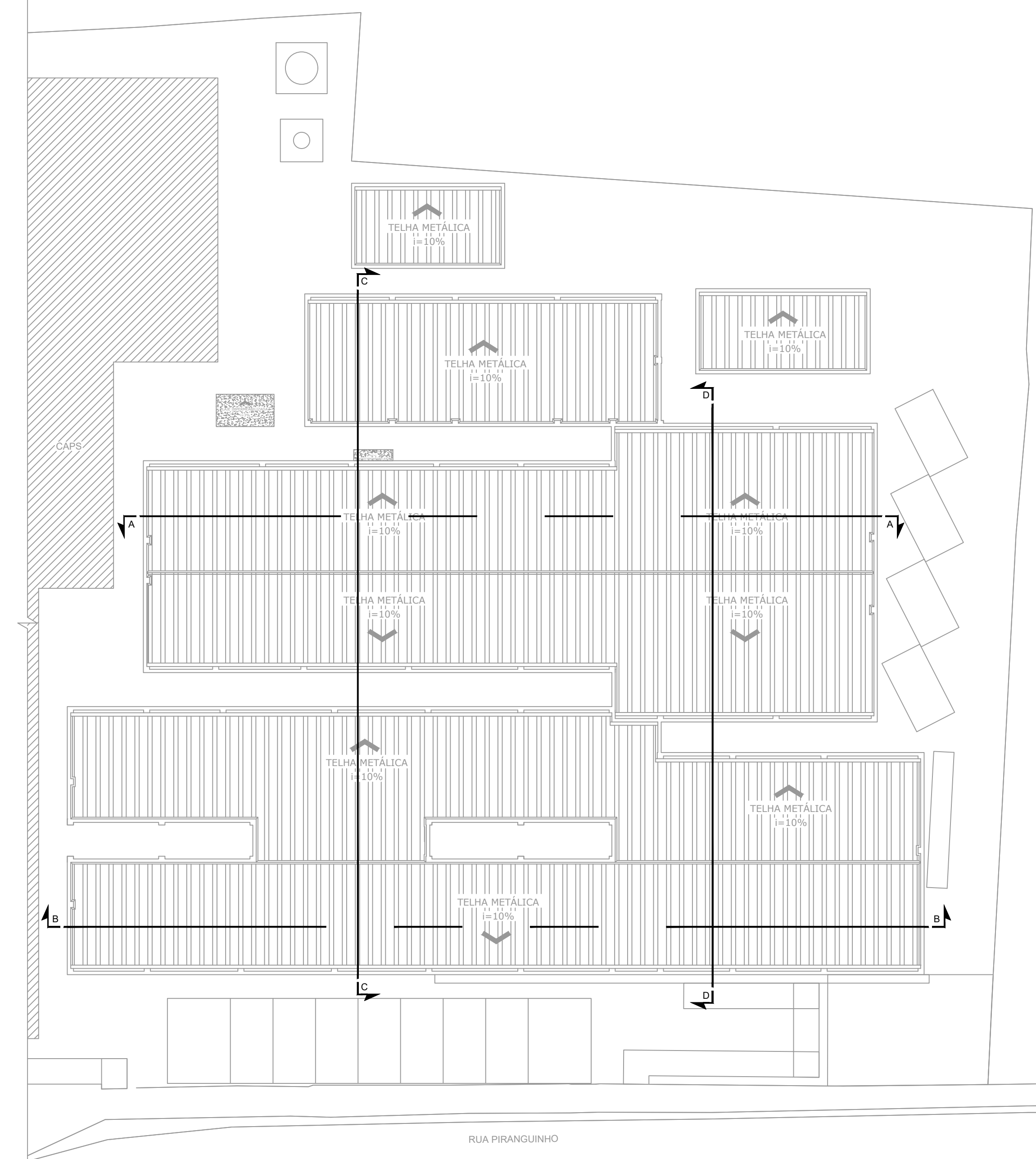
PLANTA BAIXA COBERTURA Escala: 1:200
