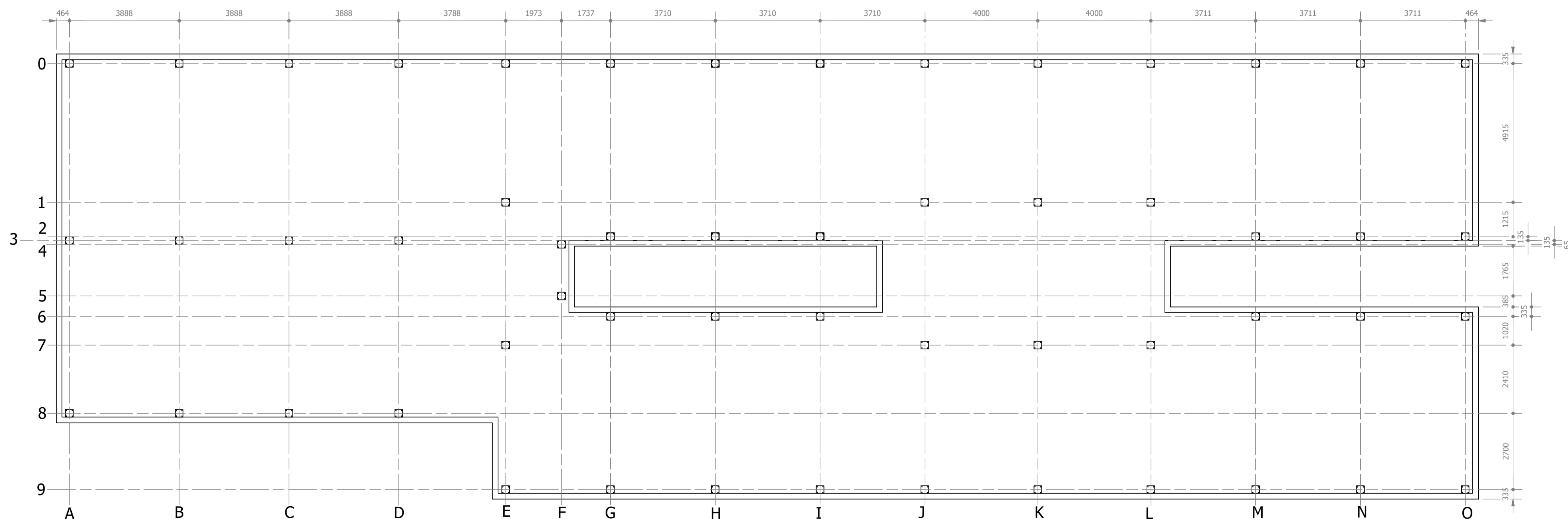
PLANTA DE LOCAÇÃO CB10 ESCALA 1 : 100
