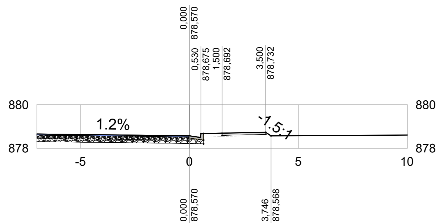
RAMO 200 - EST. 0+0,00m
