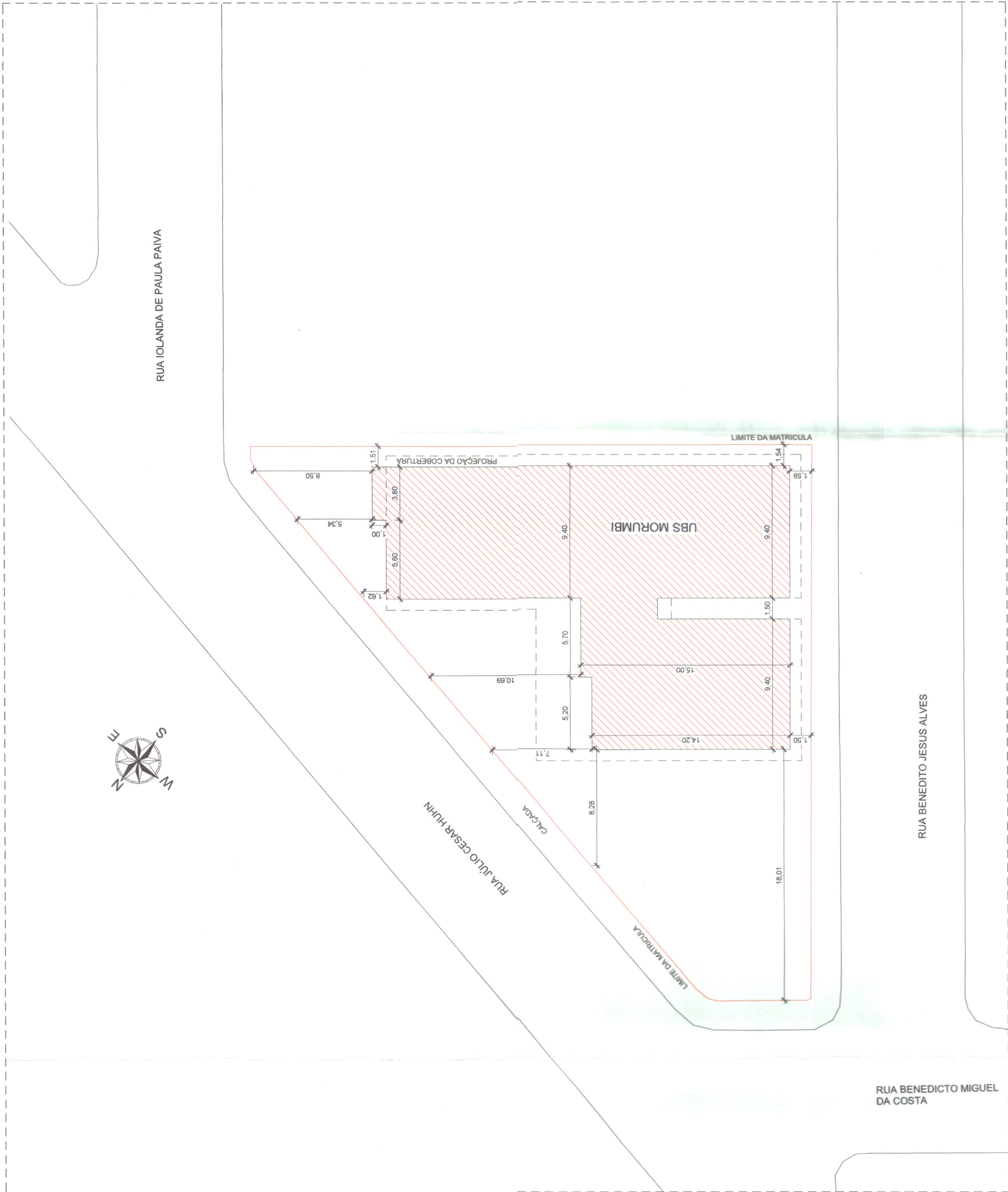
3 PLANTA DE LOCAÇÃO E SITUAÇÃO 1 : 250
