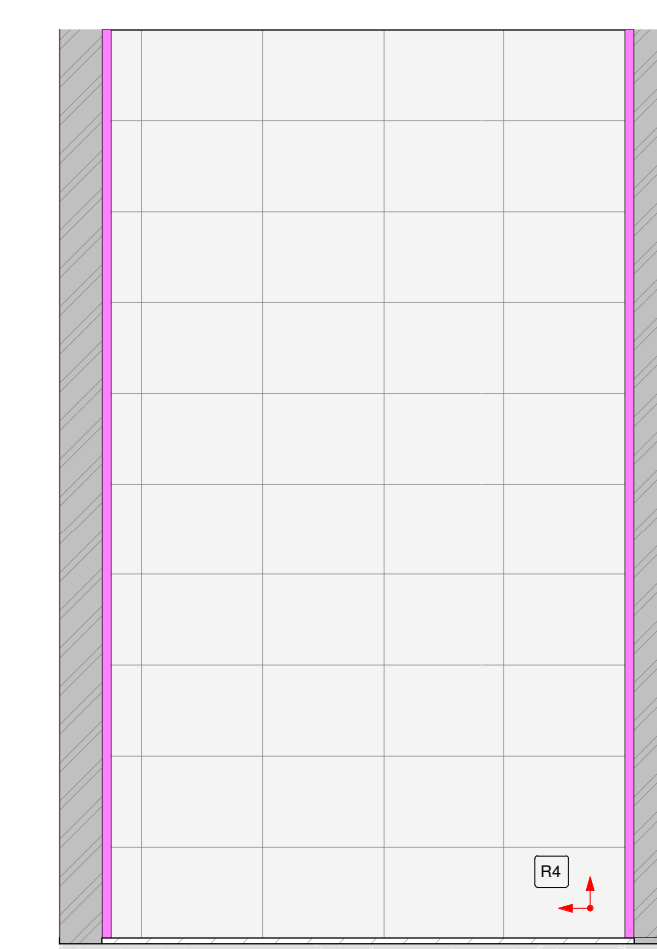
40 VISTA 2 - ABRIGO TEMP. DE RES. 1:25
