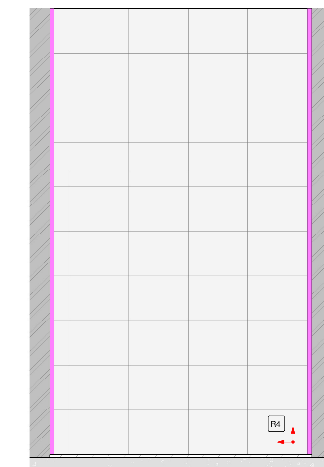
13 VISTA 1 - DML 03 1:25
