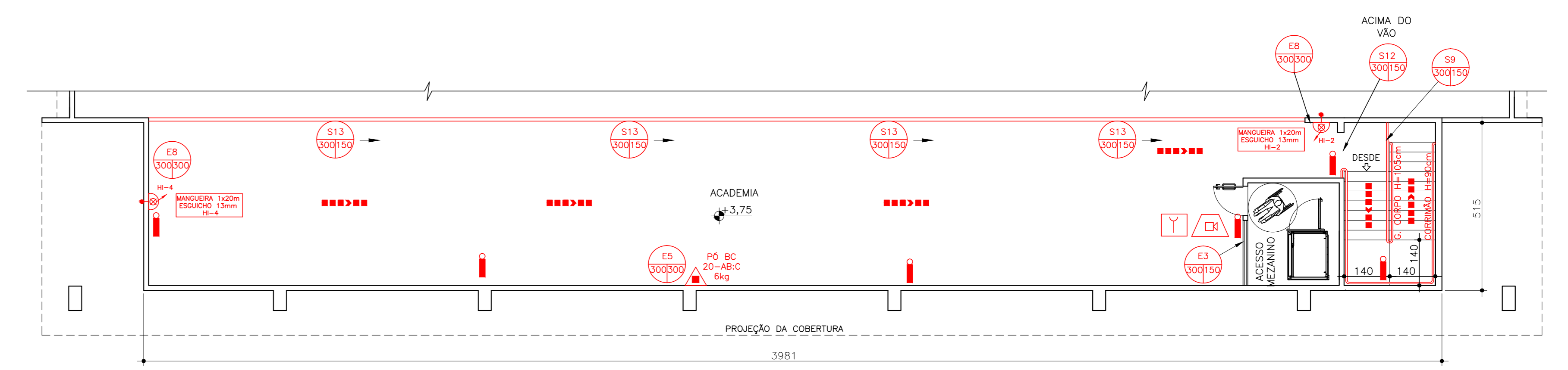
PLANTA BAIXA - GINÁSIO POLIESPORTIVO 2 - MEZANINO ÁREA: 211,00m 2 ESCALA: 1:100
