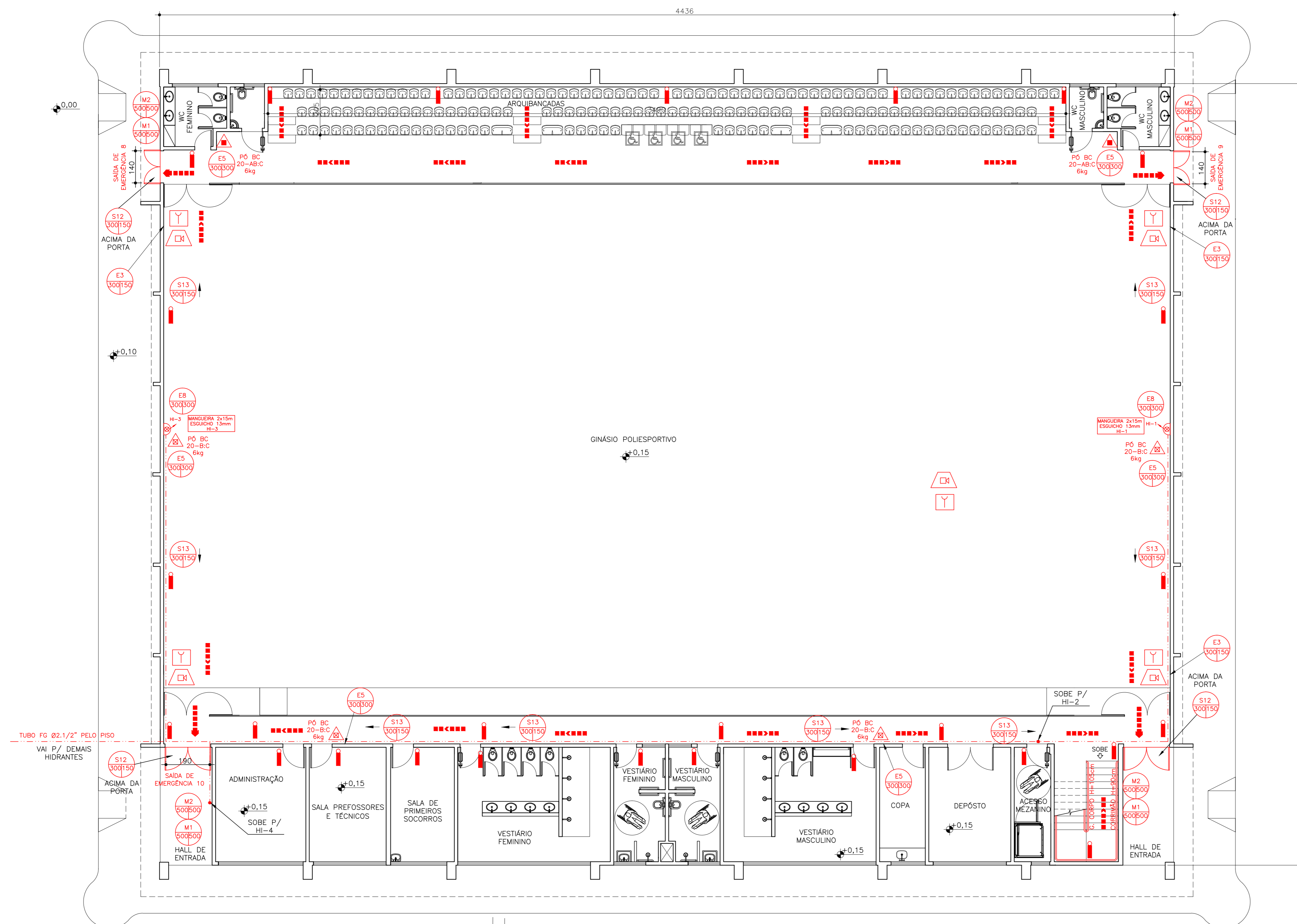
PLANTA BAIXA - GINÁSIO POLIESPORTIVO 2 - TÉRREO ÁREA: 1.675,00m 2 ESCALA: 1:100
